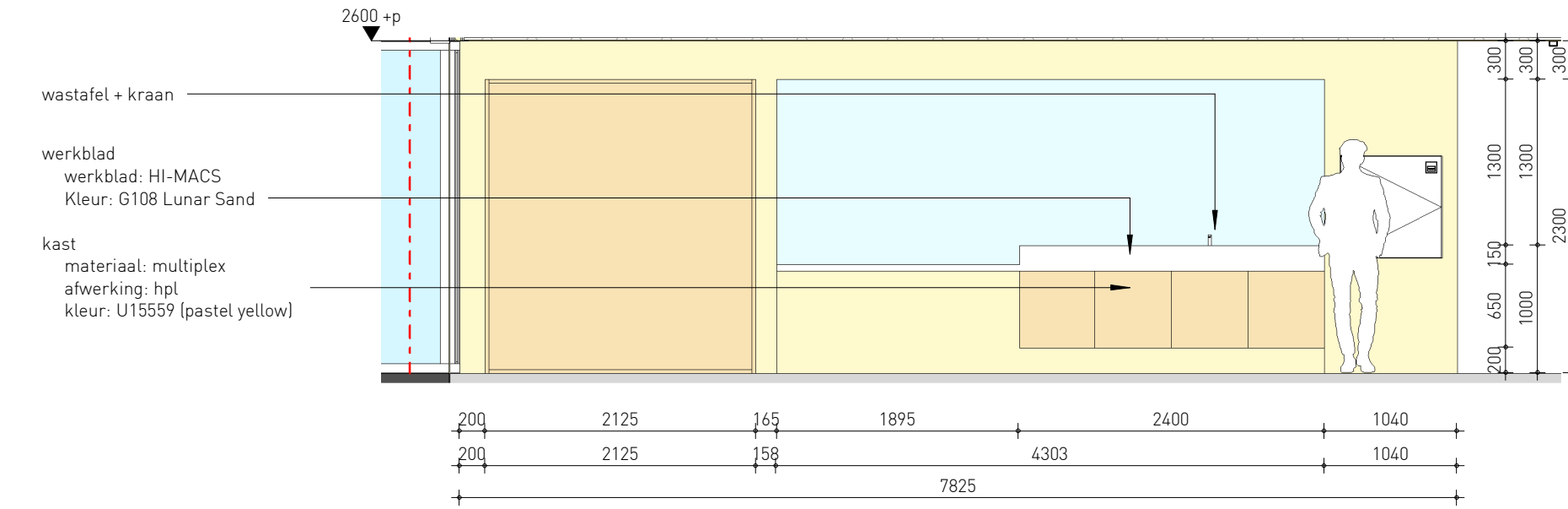
aanzicht make-up nis
