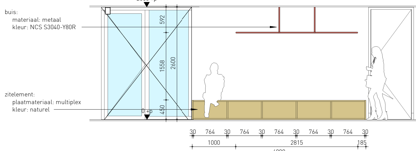
aanzicht garderobe personeel
