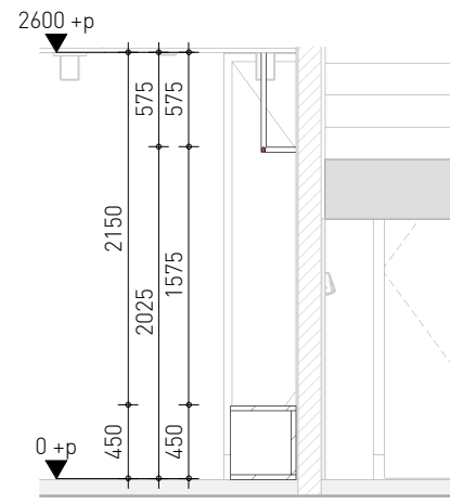
doorsnede garderobe personeel
