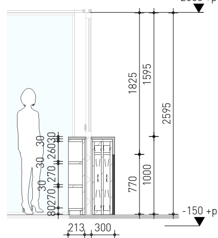
doorsnede balie
