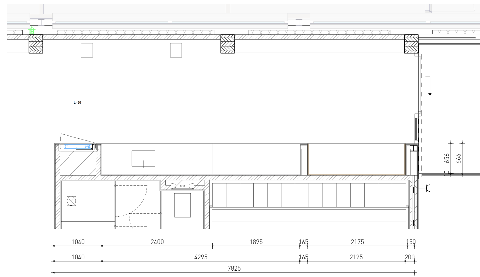
plattegrond make-up nis
