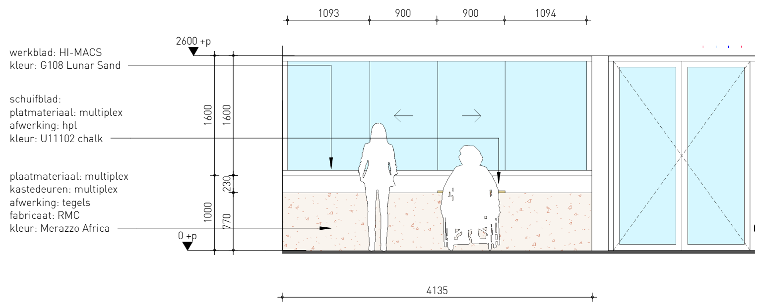
aanzicht balie
