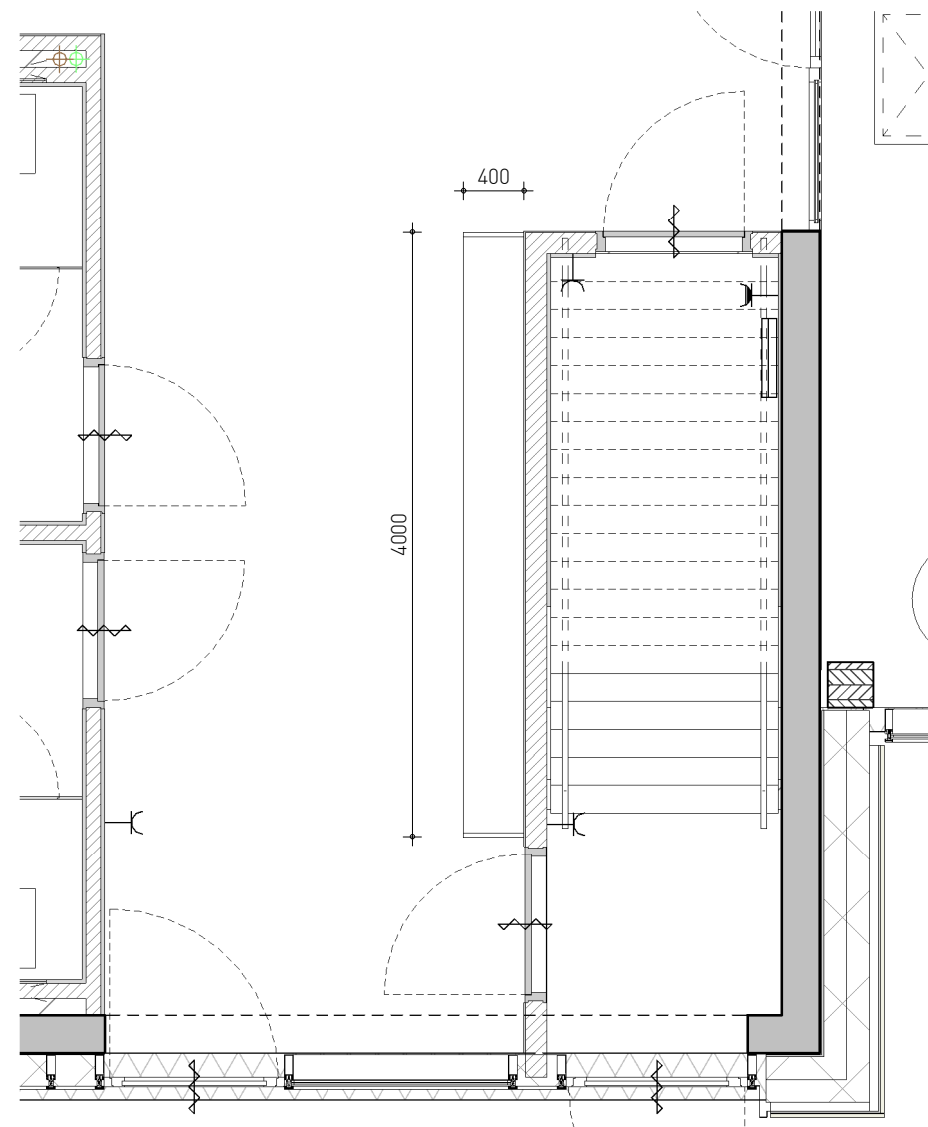
plattegrond garderobe personeel
