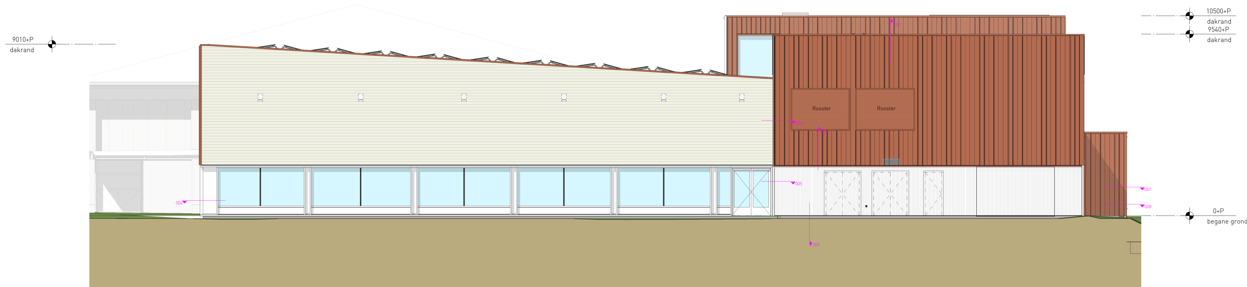
zuidgevel
