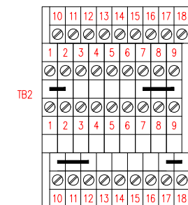
Aanzicht tekening klemmenstrook TB2 kast HF L3 T006 (Etage klem)
