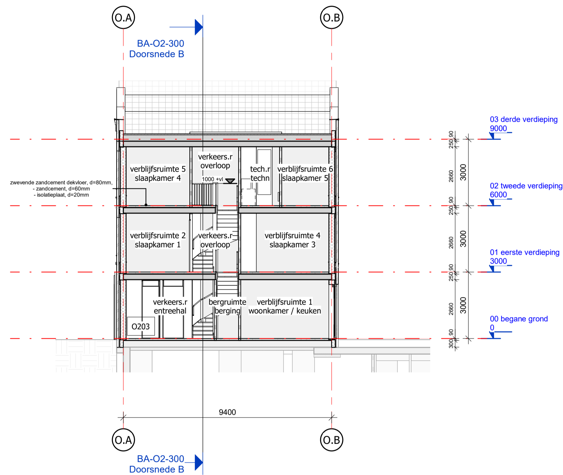
Doorsnede A schaal 1 : 100
