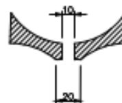
doorsnede B-B
