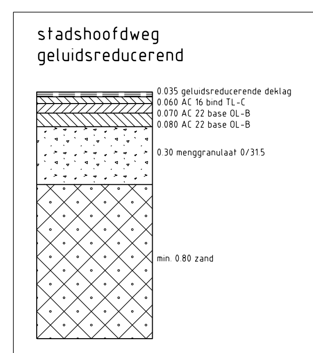
Principe nieuwe asfalt opbouw schaal: 1 : 20
