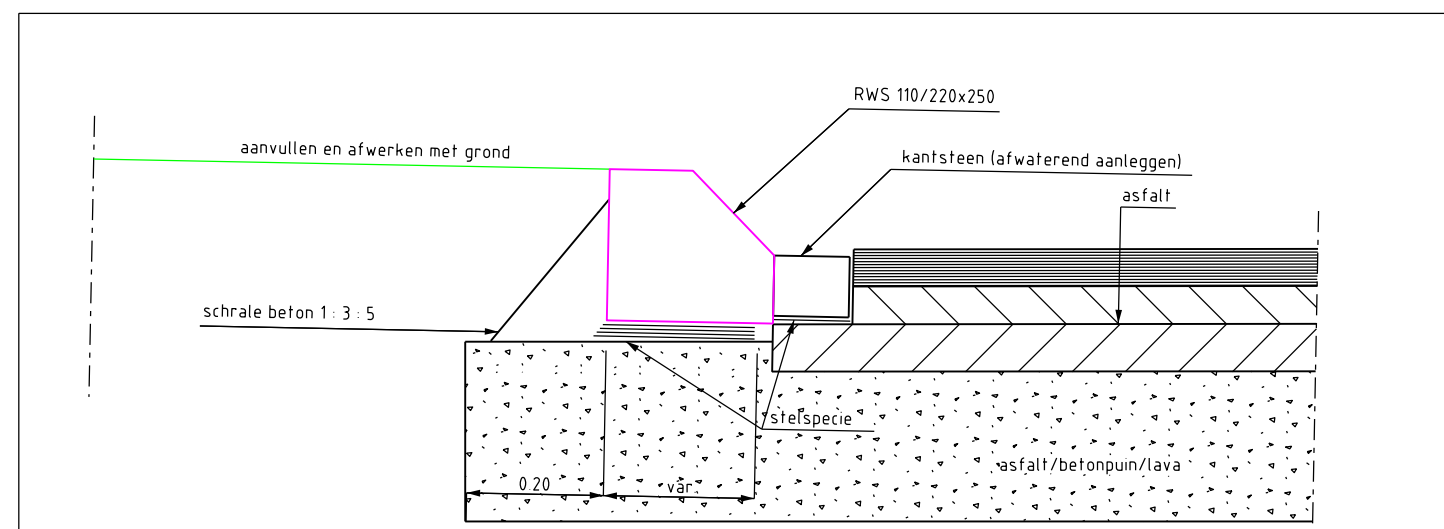
Principe trottoirband op halfverharding schaal: 1 : 10
