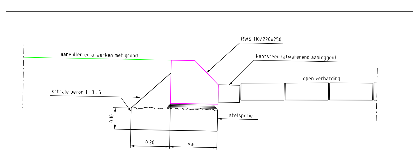
Principe trottoirband op zandbed schaal: 1 : 10
