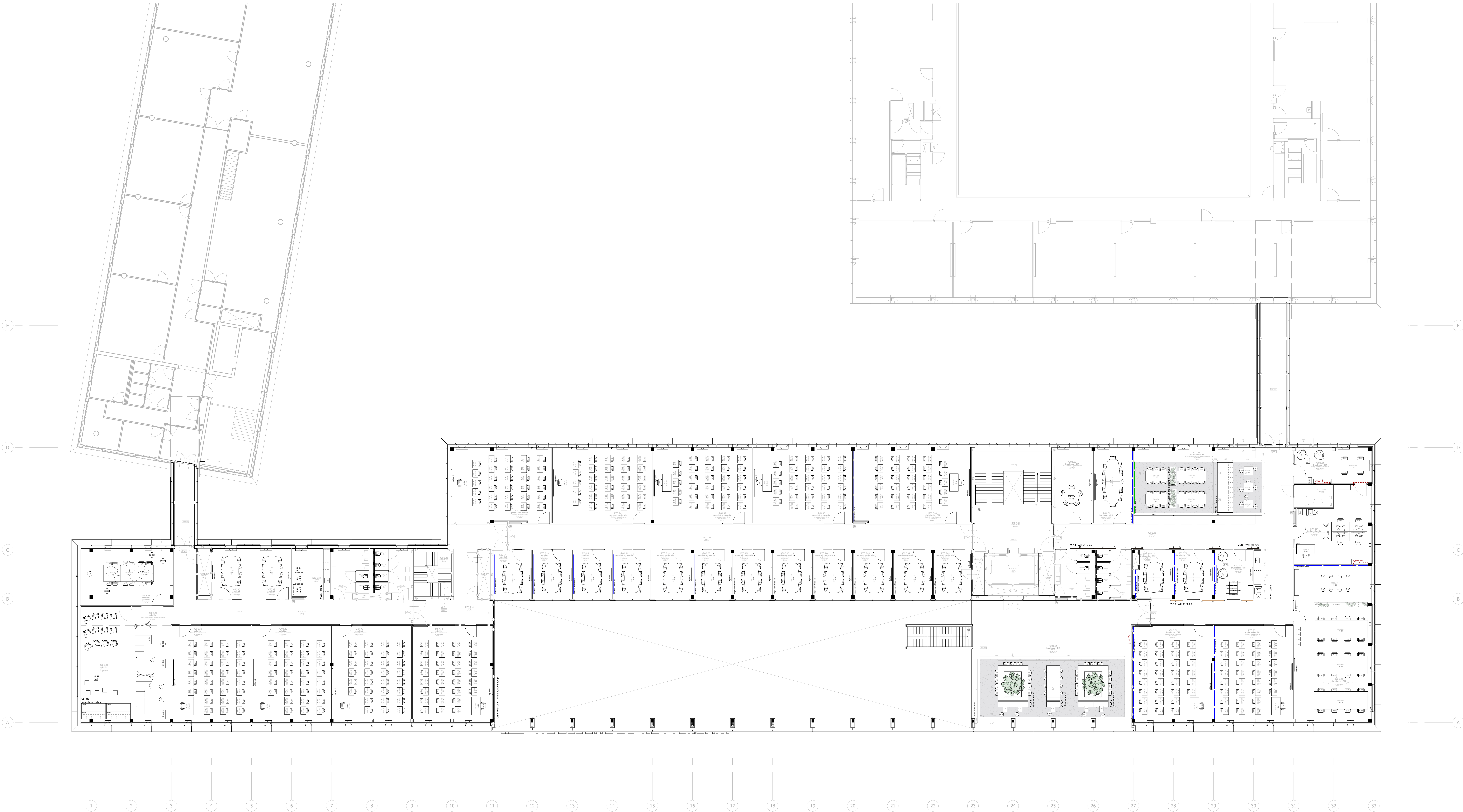
PLATTEGROND - vijfde verdieping 1:100
