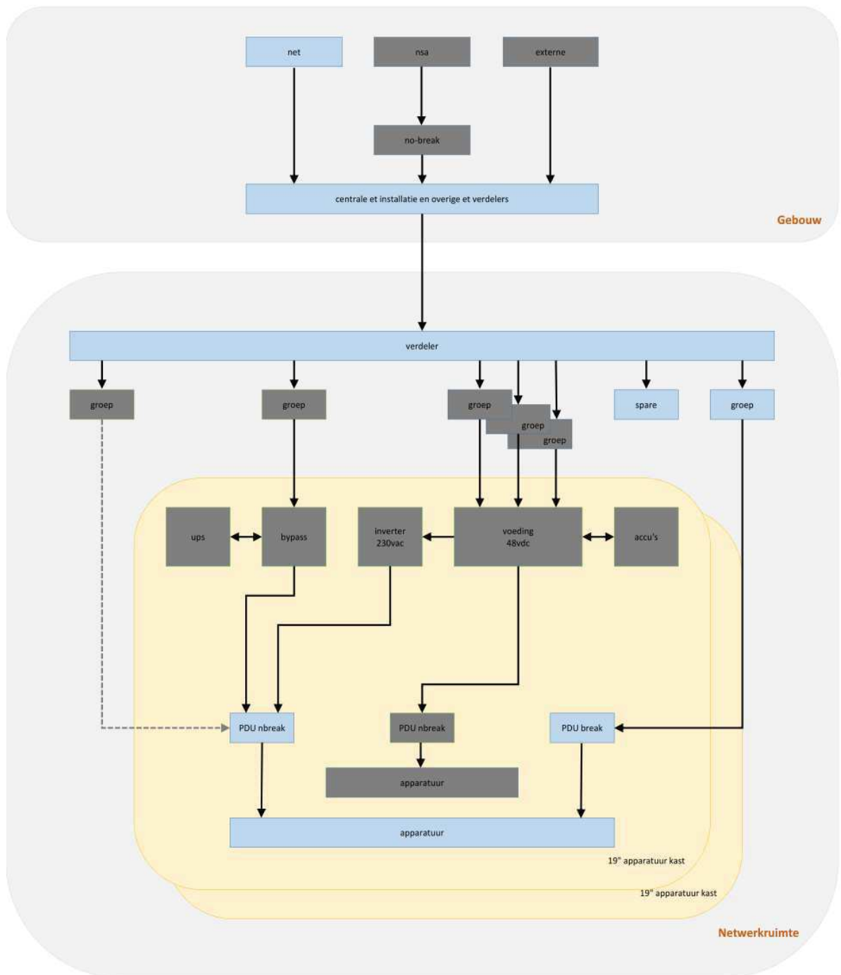
Figuur 11: Blokschema N+1 inrichting Type 3 ruimte
