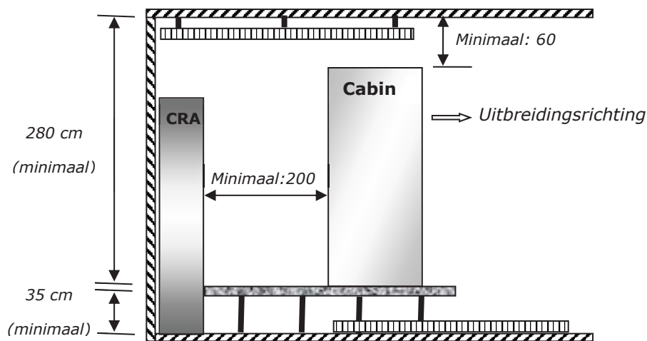
Figuur 6: Richtlijnen plafondhoogte Netwerkrumtes (2)
