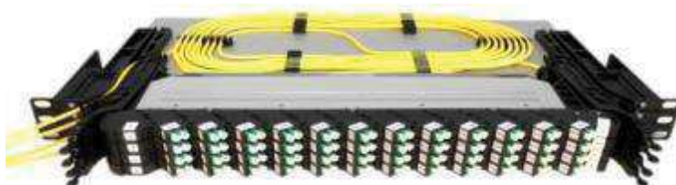
Figuur 27: FLODF met pre-terminated patch-cassettes en overlengte
