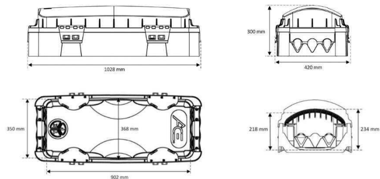
Figuur 15. Handhole voor Local Tail (type 1 – ACE-TKF)
