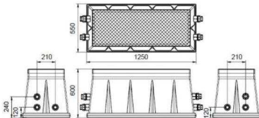
Figuur 17. Handhole voor MER (type - Zweva Z6P)
