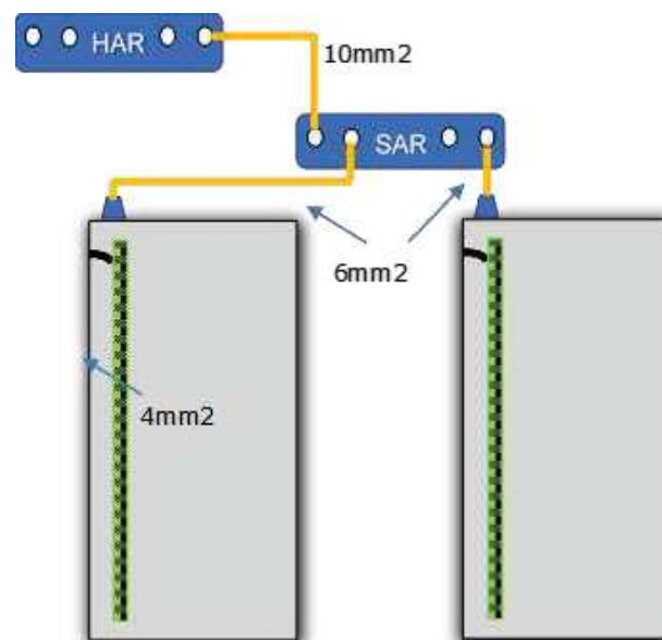
Figuur 3: Aardingsprincipe cabinets met uitsluitend 230VAC
