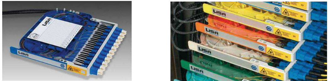
Figuur 10: H&S LISA Fibertrays
