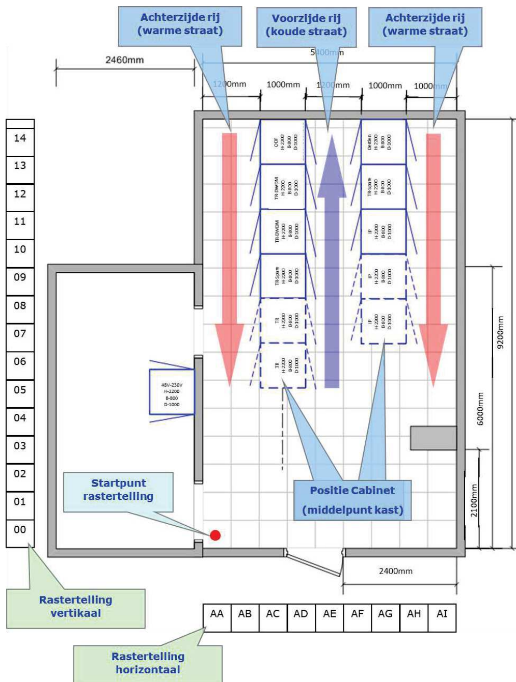
Figuur 1: Voorbeeld rastertelling vloerplan
