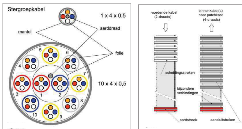
Figuur 3: Principe indeling stergroepkabel en afwerking op LSA+
