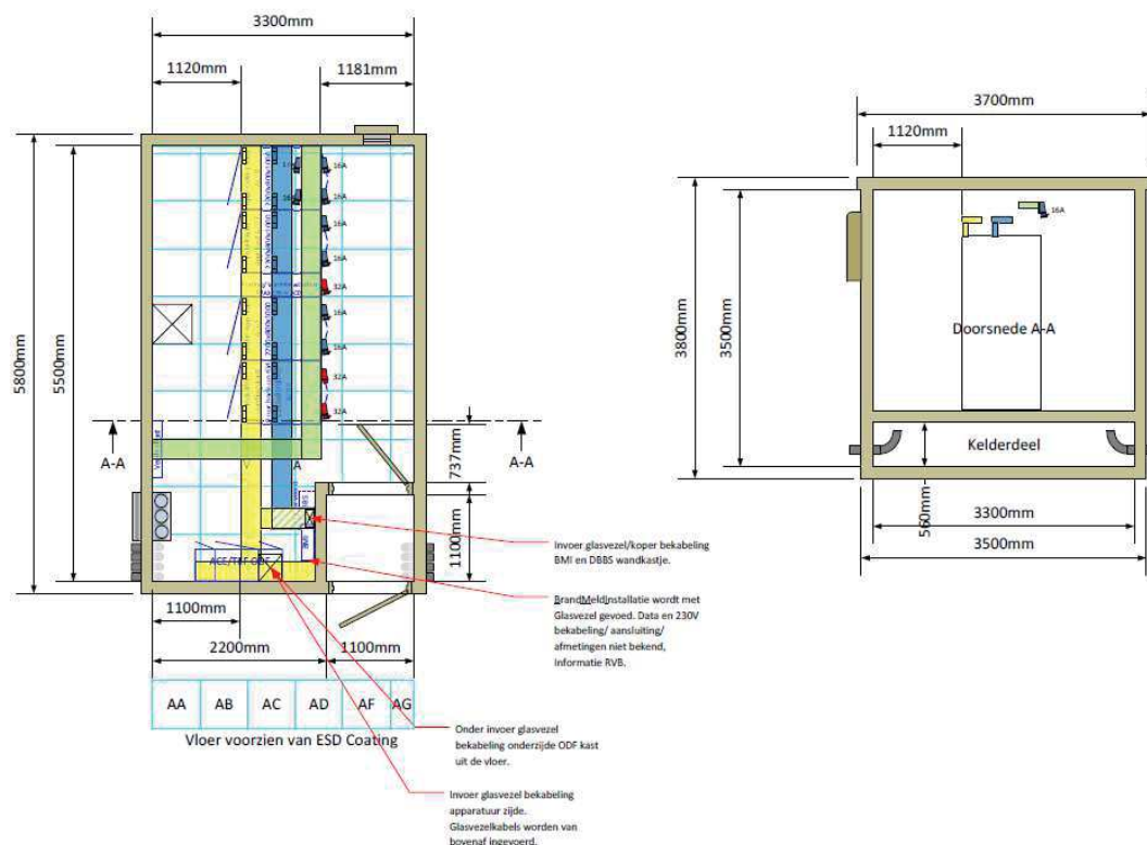
Figuur 11: Inrichting POP
