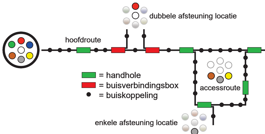
Figuur 1: Microduct infrastructuur
