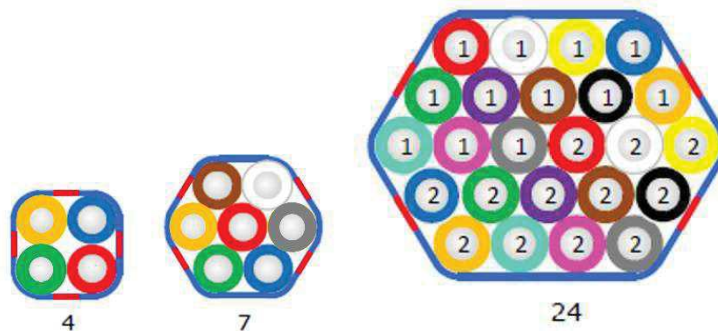
Figuur 18. Samenstelling en kleurcodering DB-buis Emtelle
