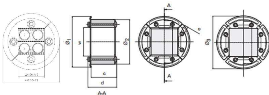
Figuur 20. Roxtec invoerblok
