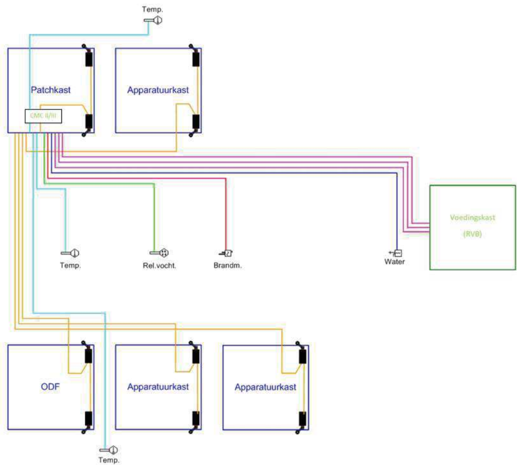
Figuur 2: Voorbeeld monitoring oplossing Type 2 Netwerkrumte
