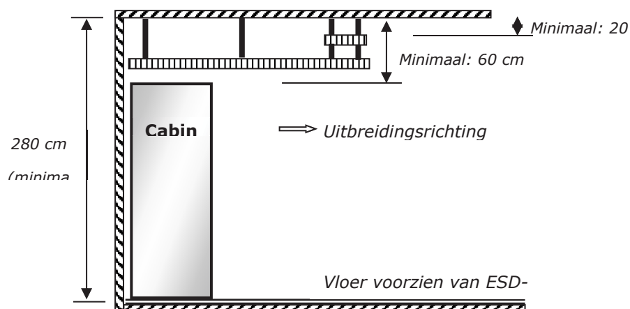
Figuur 5: Richtlijnen plafondhoogte Netwerkrumtes (1)
