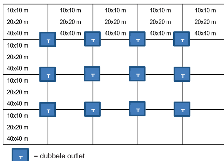
Figuur 14: Principeschema raster tbv WiFi-outlets
