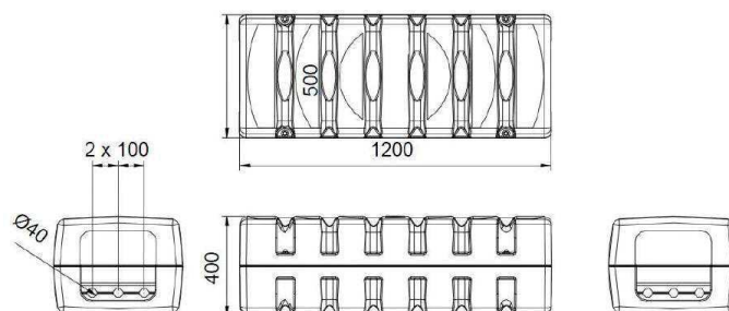
Figuur 16. Handhole voor Local Tail (type 2 – Zweva HHZ)
