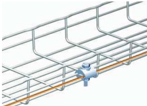
Figuur 5: Voorbeeld galvanische koppeling aarding draadgoot
