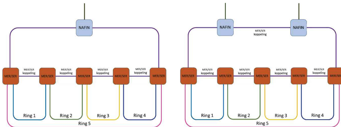
Figuur 14. LPI-glasvezelinfra, >2 ringen 1 NAFIN opstijggpunt
