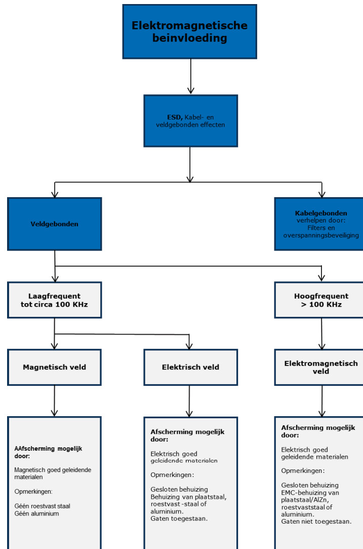
Figuur 11: Flowchart technische maatregelen Elektromagnetische beïnvloeding
