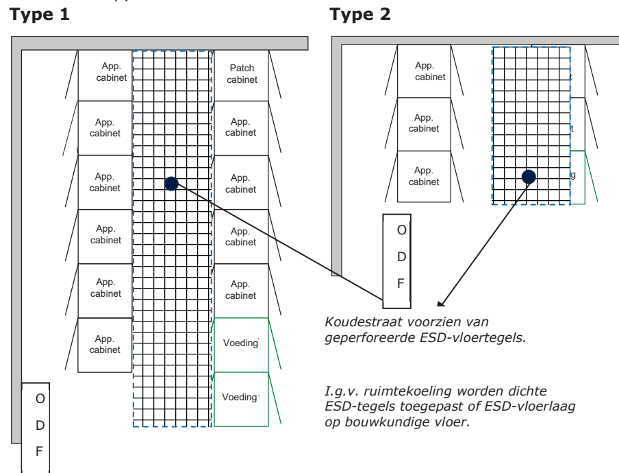
Figuur 3: Voorbeeld standaardinrichting type 1 en type 2 netwerkrumte
