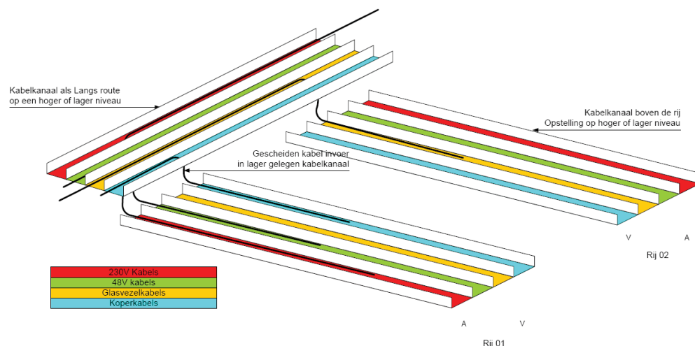
Figuur 8: Scheiding bekabeling installatiedelen draadgootoplossing
