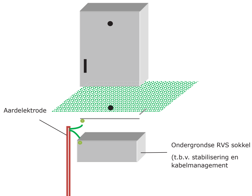
Figuur 3: Principe overzicht plaatsing Outdoor Cabinet
