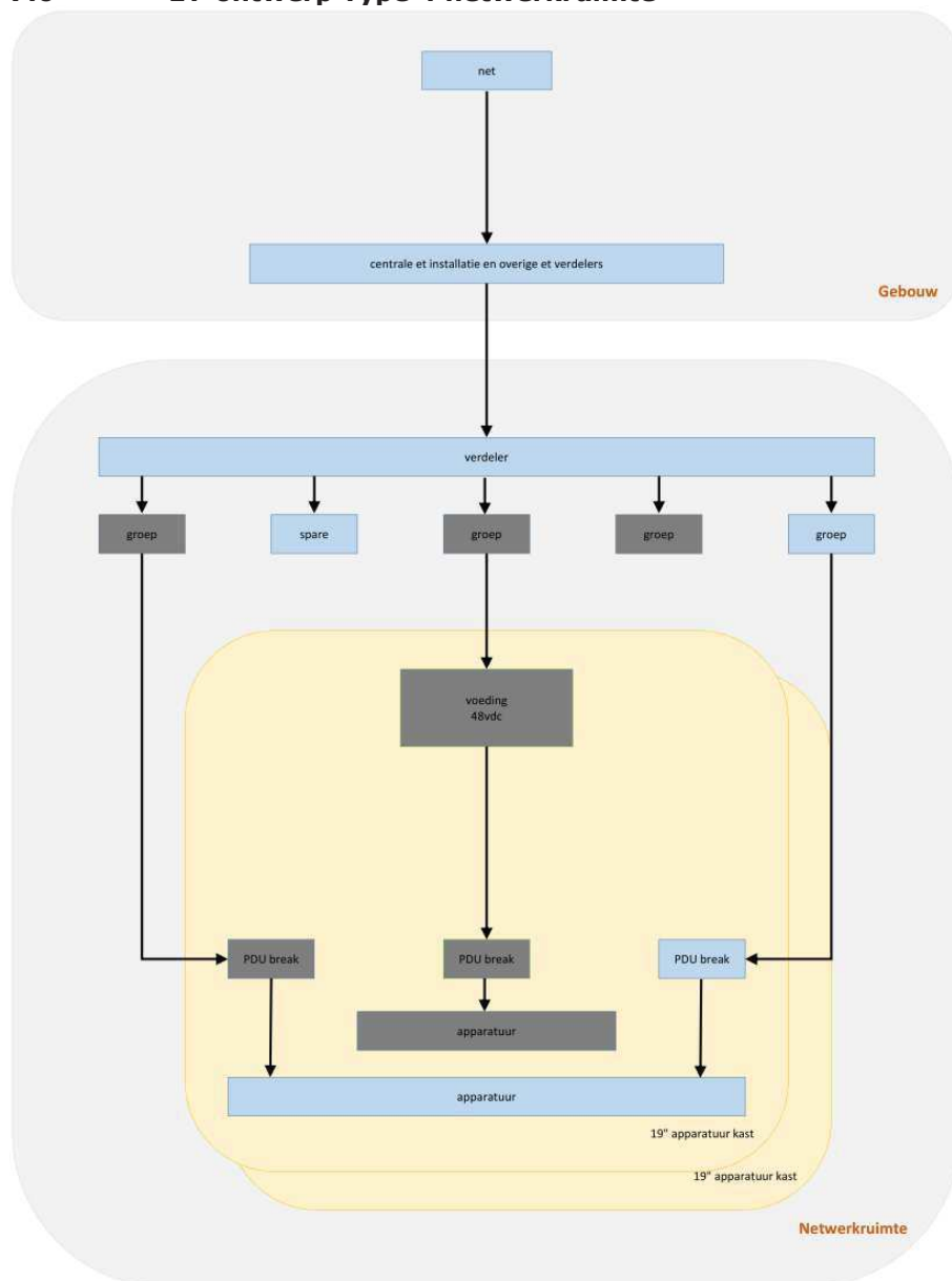
Figuur 12: Blokschema N inrichting Type 4 ruimte
