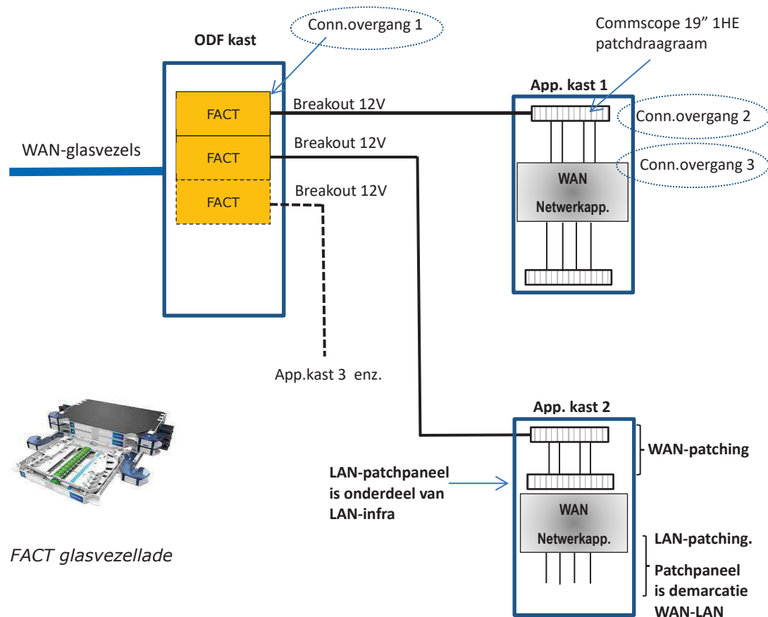
Figuur 12: Schematische weergave 3-connector model NAFIN-WAN
