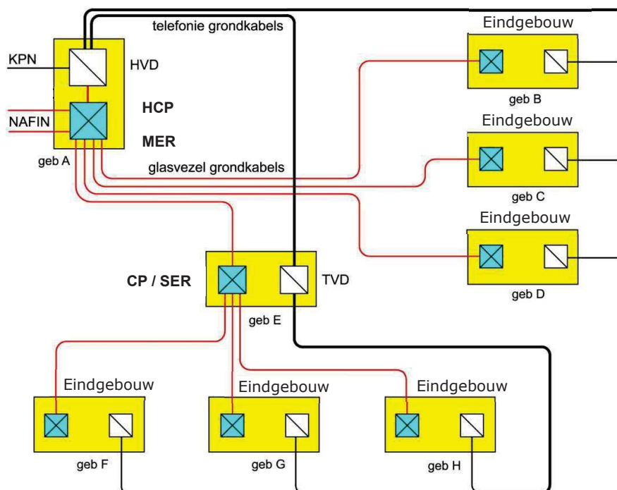
Figuur 2: Voorbeeld infrastructuur op Defensieobject
