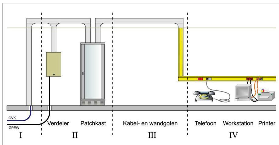
Figuur 1: Schematische weergave Opbouw LPI
