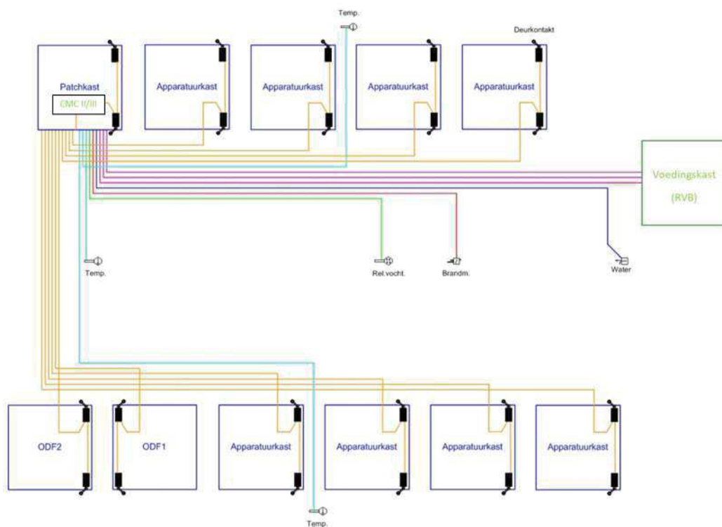
Figuur 1: Voorbeeld monitoring oplossing Type 1 Netwerkrumte
