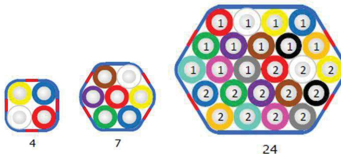
Figuur 19. Kleurcodering DB-buis (type 2 -Prysmium)
