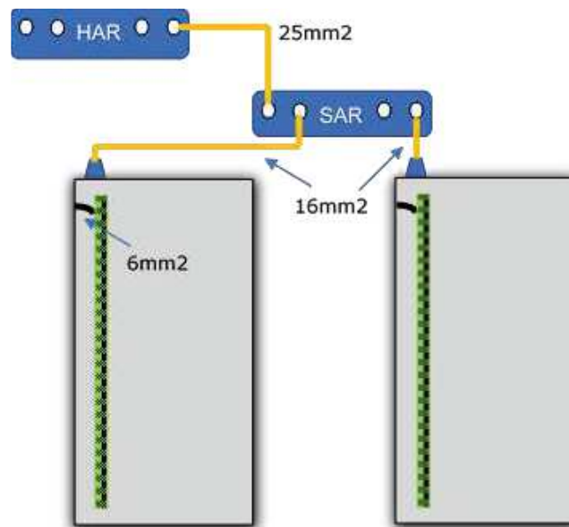
Figuur 2: Aardingsprincipe cabinets met uitsluitend -48VDC
