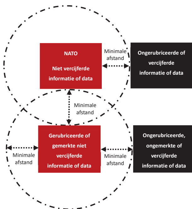
Figuur 6: ROOD-ROOD scheiding
