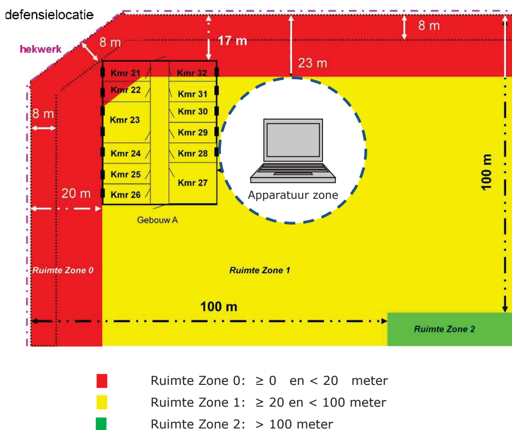
Figuur 8: Schematische weergave apparatuur zonering
