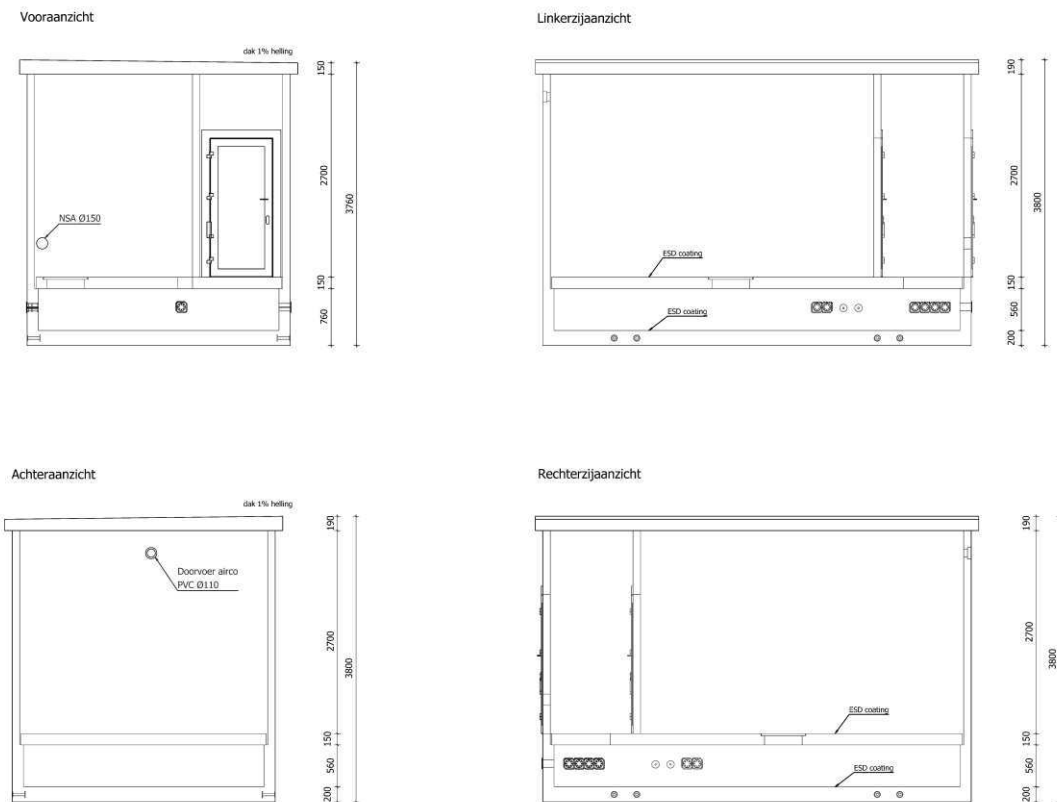
Figuur 10: Bouwkundige maatvoering POP
