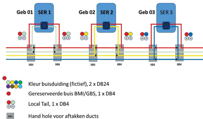
Figuur 11. Principeschema aftakkingen Local Tails per gebouw
