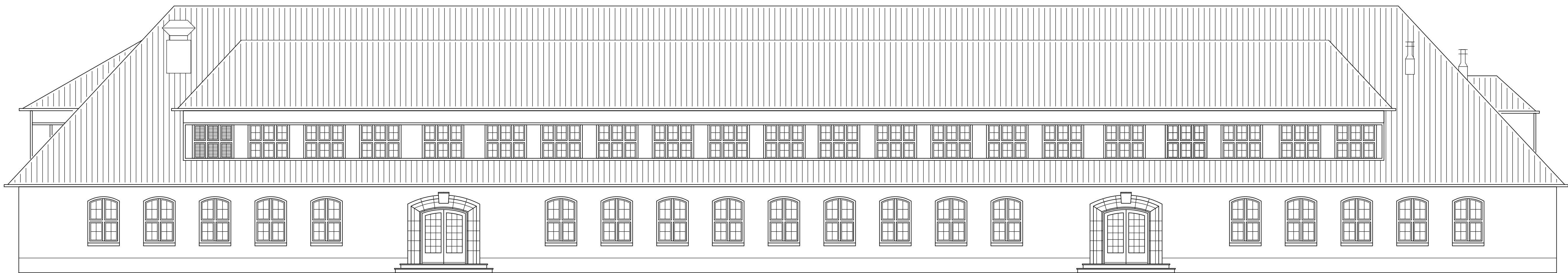
ZUIDGEVEL
