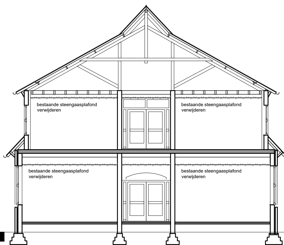
DWARSDOORSNEDE
