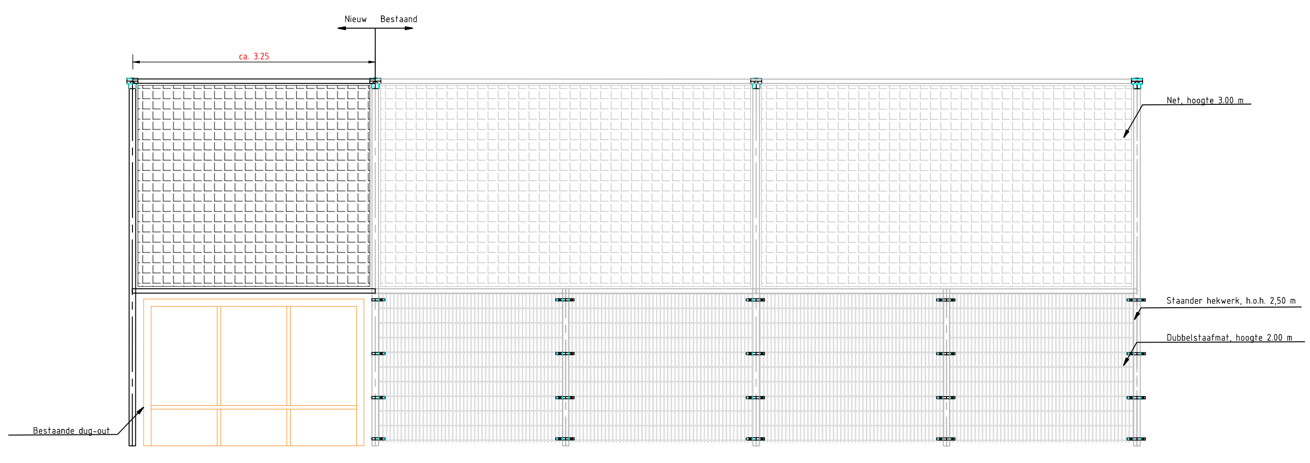
Voorraanzicht B - Uitbreiding ballenvanger Schaal 1 : 50
