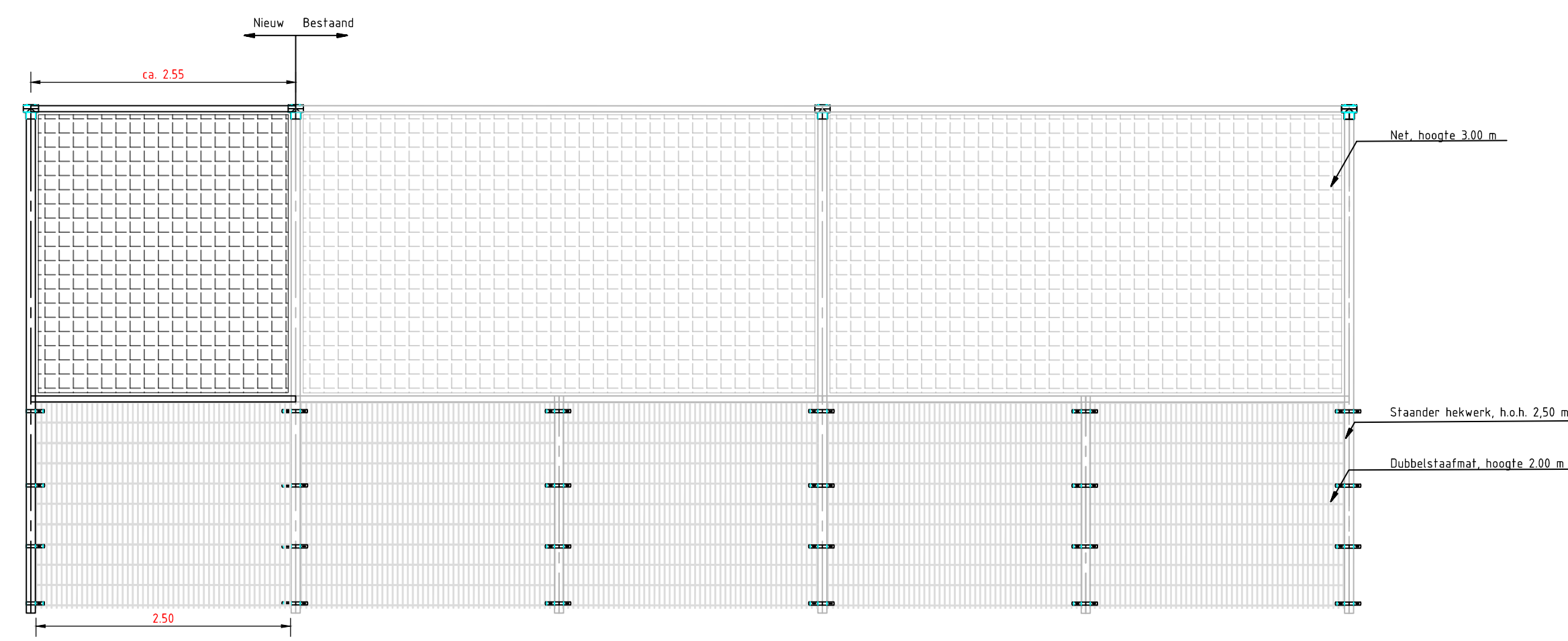
Voorraanzicht A - Uitbreiding ballenvanger Schaal 1 : 50
