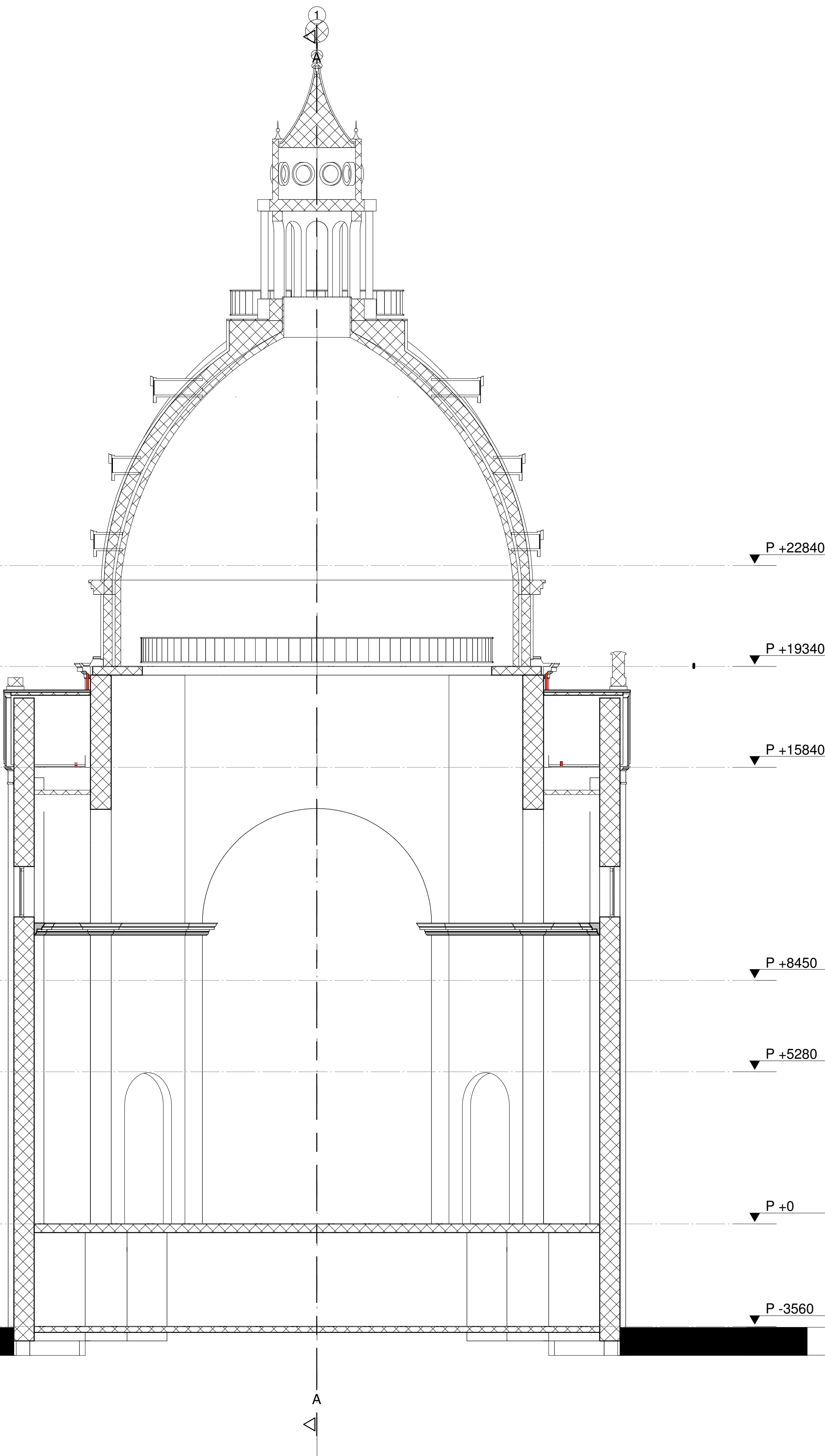
doorsnede B-B
