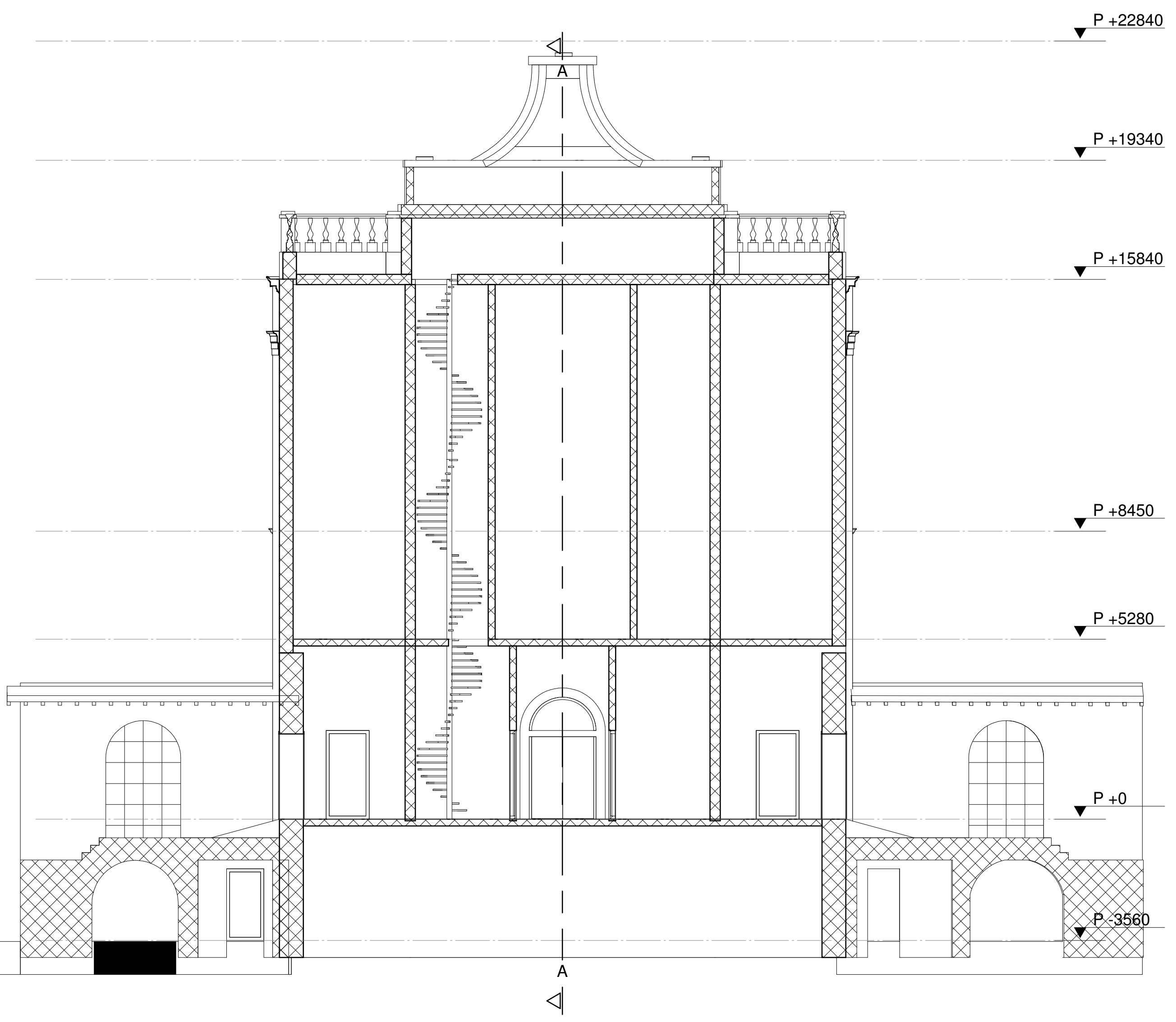
doorsnede C-C
