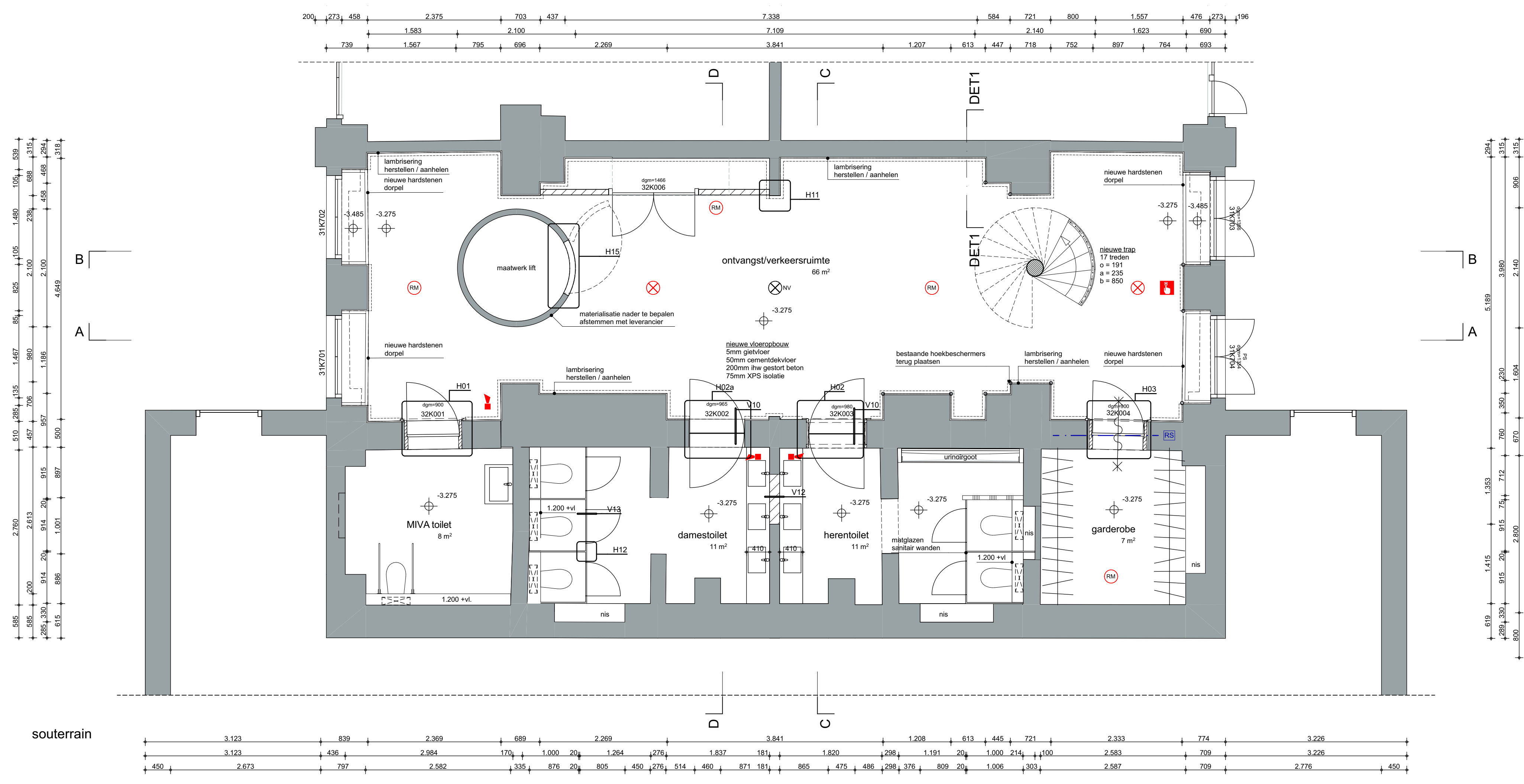
begane grond
