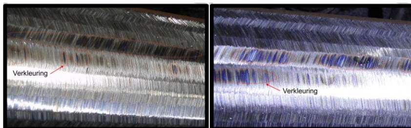
FIGUUR 4: VOORBEELDEN VAN DIRECTE AFKEUR. ZWARTE SLIJPGROEVEN (LINKS), HELDER BLAUW IN SLIJPGROEVEN (RECHTS).
