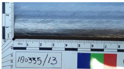
FIG 3: BEWERKT OPPERVLAKE MET TOEGESTANE LICHT VERKLEURING (ZELFDE ALS IN FIG 2)
