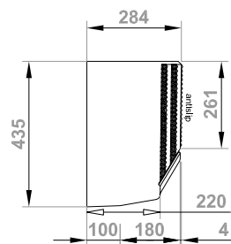
Zijaanzicht links
