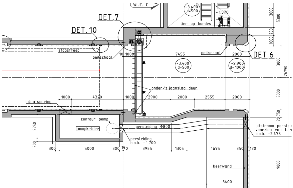
Afbeelding 2-3: Doorsnede pompkelder en uitstroomleiding.*
