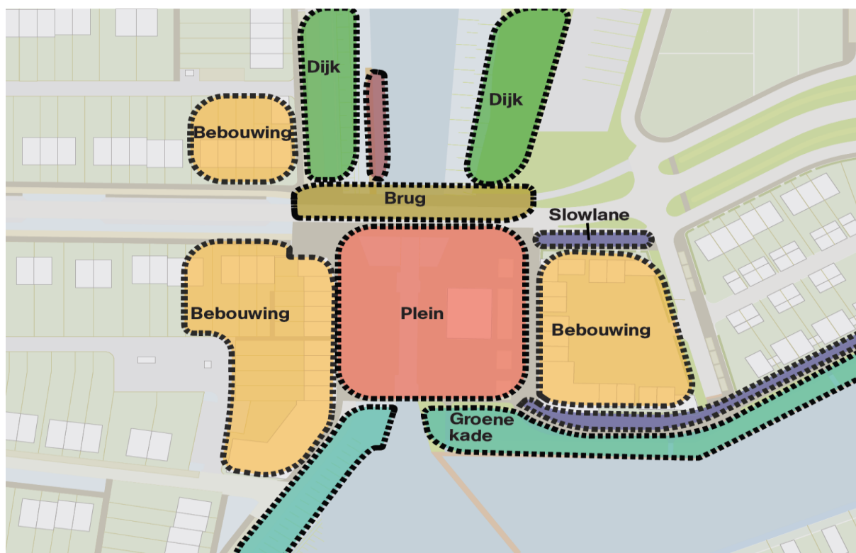
Afbeelding 2-4: Ontwerp LAOS locatie beweegbare Sluisbrug en omgeving.*
