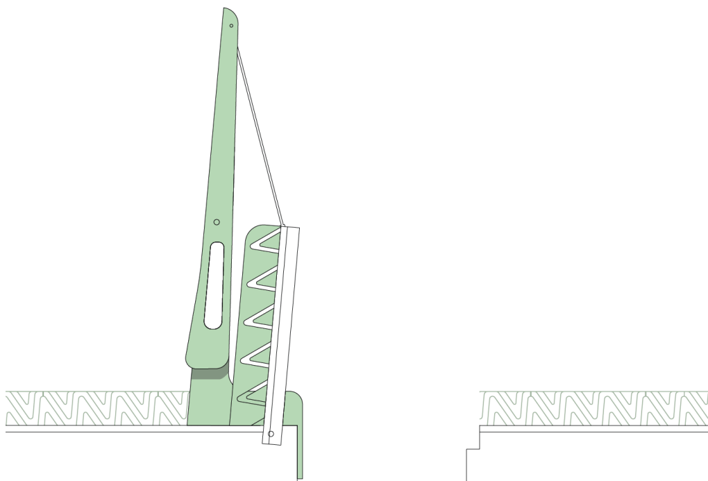
Afbeelding 2-6: Ontwerp LAOS, zijaanzicht geopende brug.*
