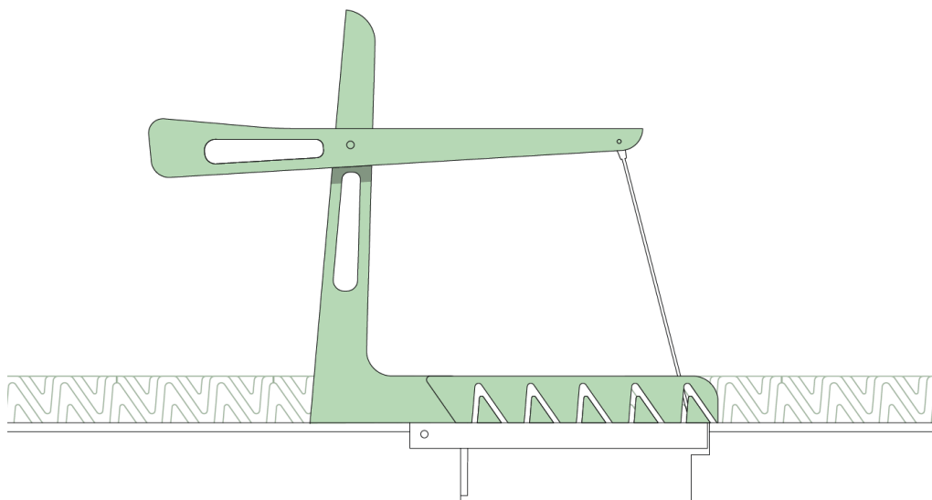
Afbeelding 2-5: Ontwerp LAOS, zijaanzicht gesloten brug.*
