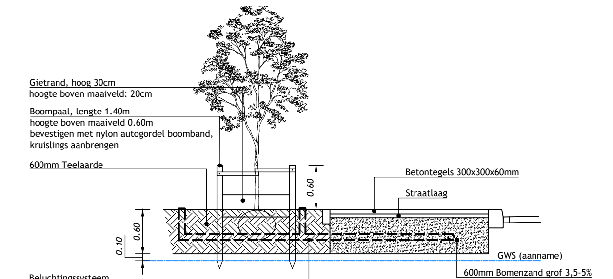
Dwarsprofiel 1 Schaal 1:50
