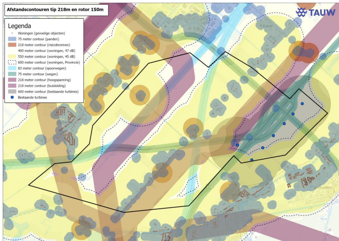
Figuur 11: Diverse afstandscontouren voor een windturbine met tiphoogte 218m en rotor 150m ten opzichte van verschillende functies, Bron data Pondera
