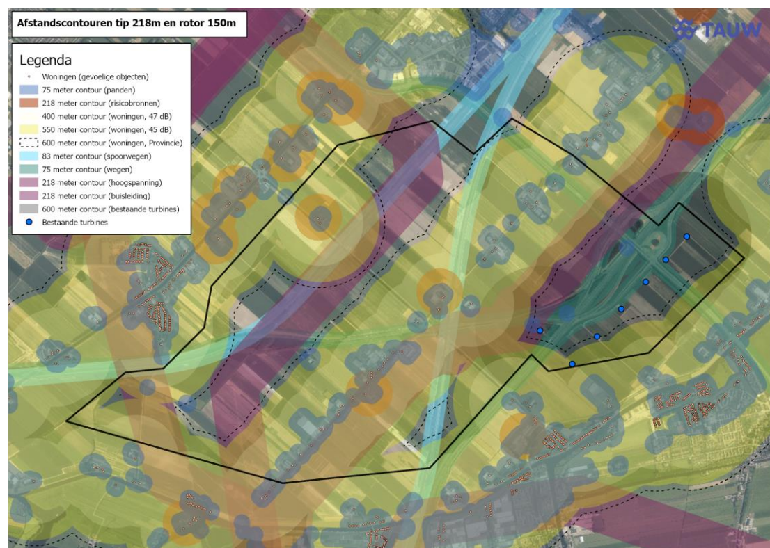
Figuur: Diverse afstandscontouren voor een windturbine met tiphoogte 218m en rotor 150m ten opzichte van verschillende functies op luchtfoto, Bron data Pondera
