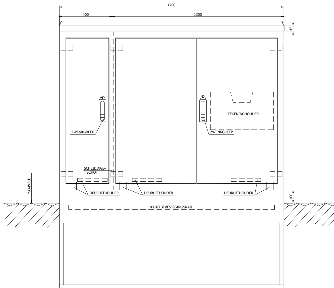
VOORAANZICHT
