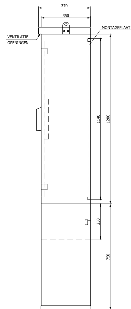
ZIJAAANZICHT RECHTS
