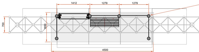
Bovenaanzicht
