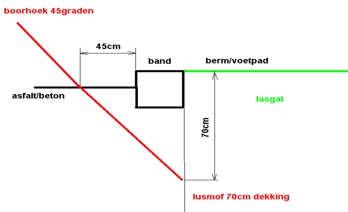
Schema aanbrengen boorgat detectielussen
