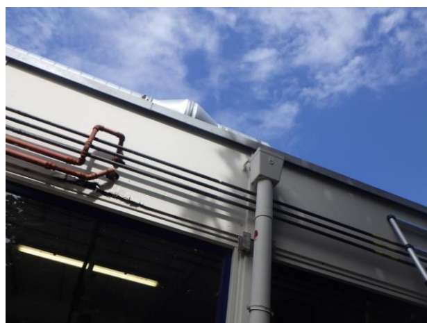
Hemelwaterafvoer van pvc
