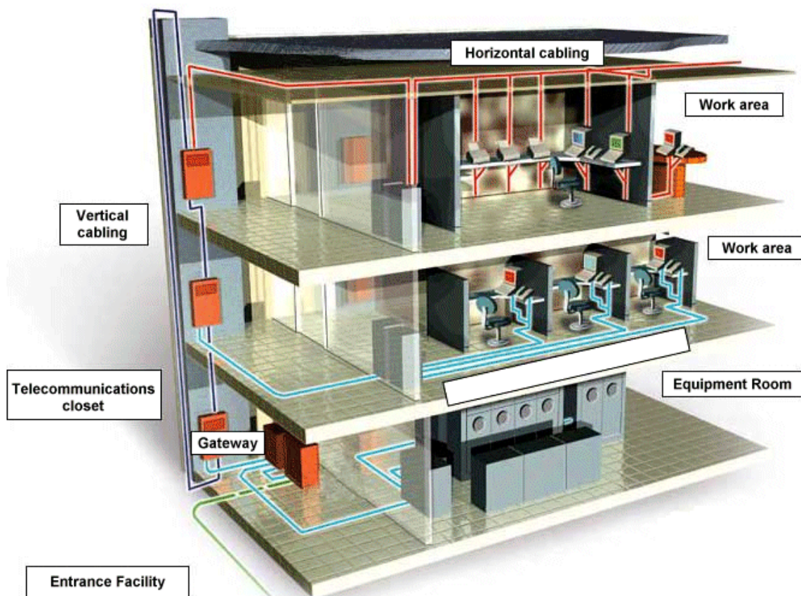
Figuur 1: Opbouw data bekabelings systeem.
