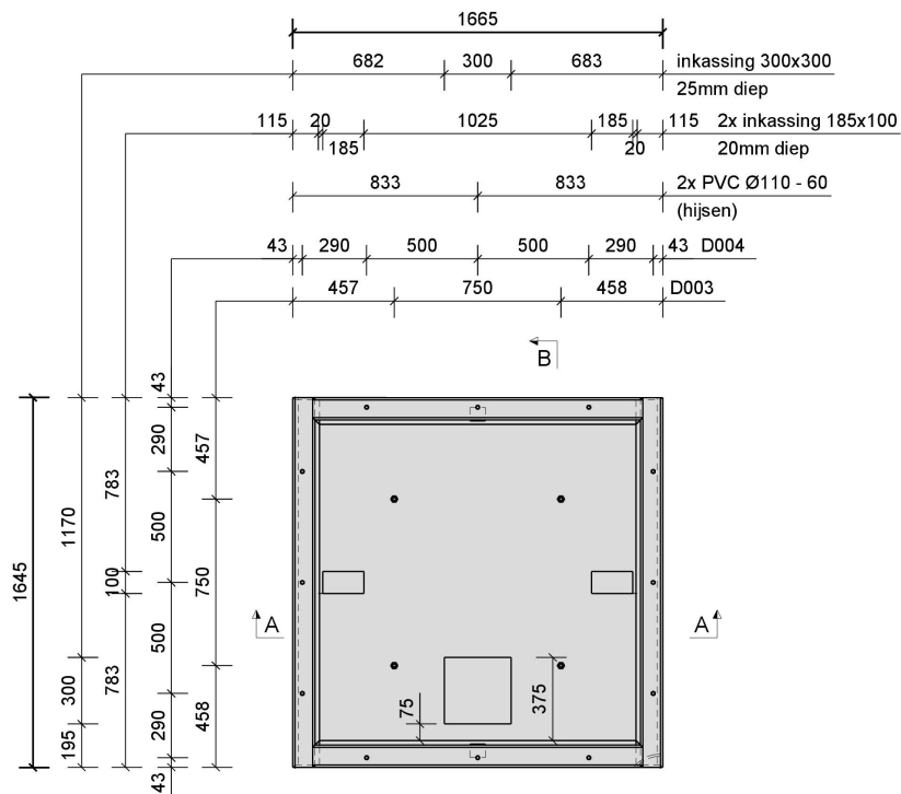
Bovenaanzicht 1:25
