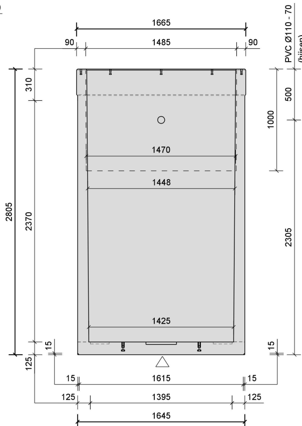
Doorsnede A 1:25
