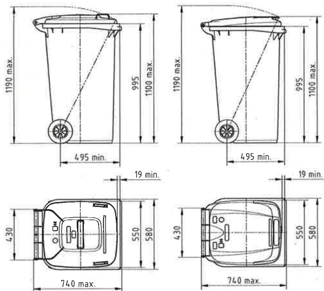
Standaarddeksel
