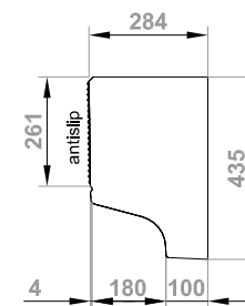
Zijaanzicht rechts
