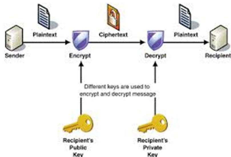
Afbeelding 1: Asymmetrische encryptie
