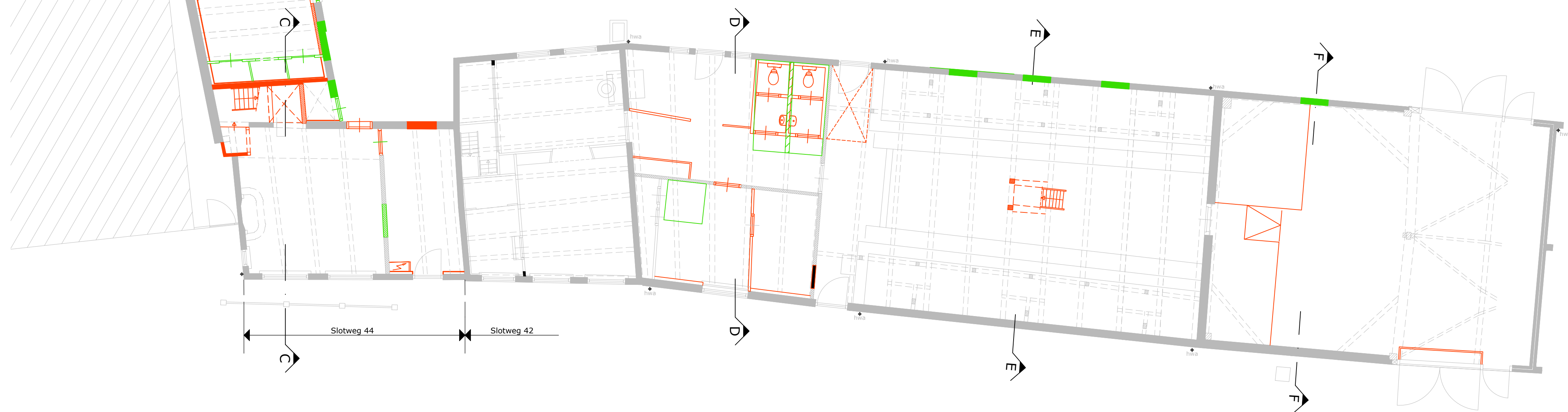
BEGANE GROND
