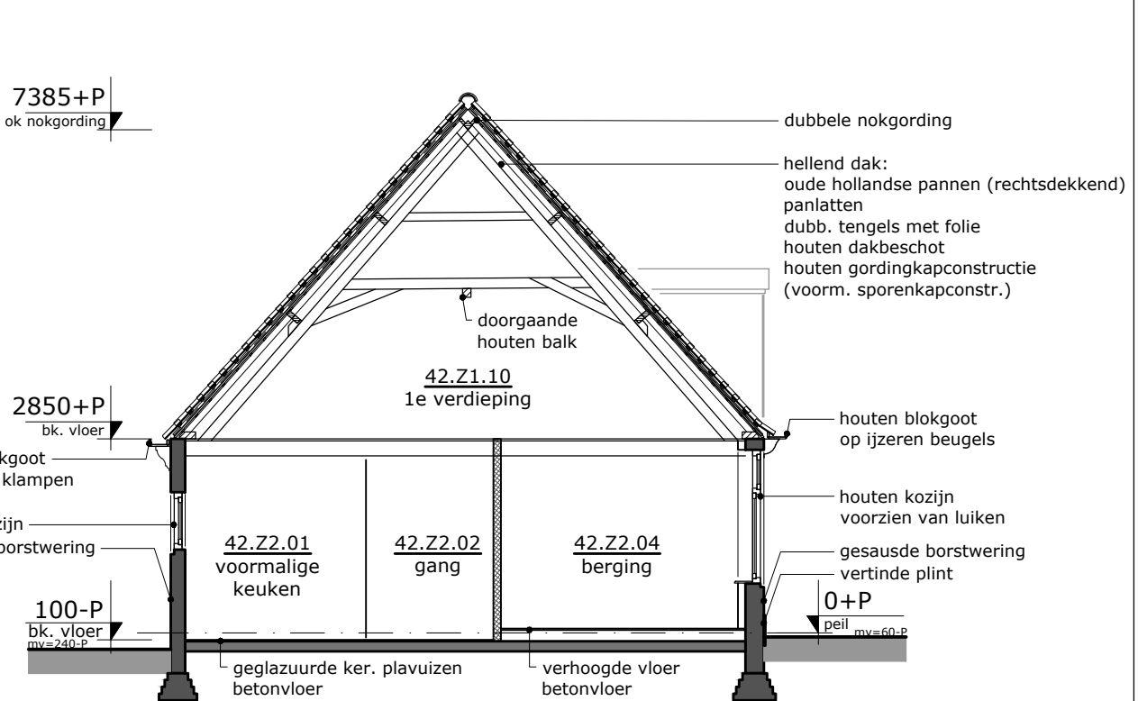
DOORSNEDE D bouwdeel 42_Z2 doorsnede van hoofdspant
