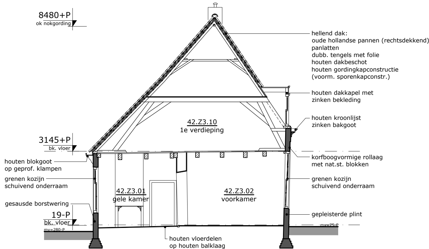
DOORSNEDE G bouwdeel 42_Z3 doorsnede van hoofdspant
