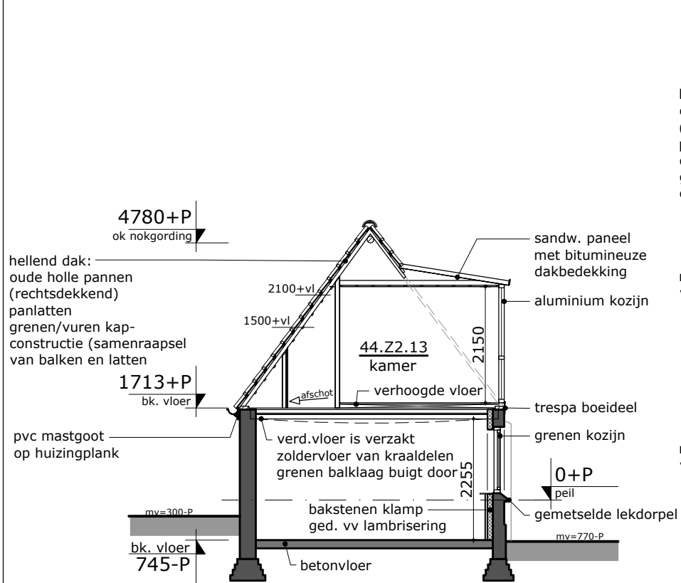
DOORSNEDE A bouwdeel 44_Z2
