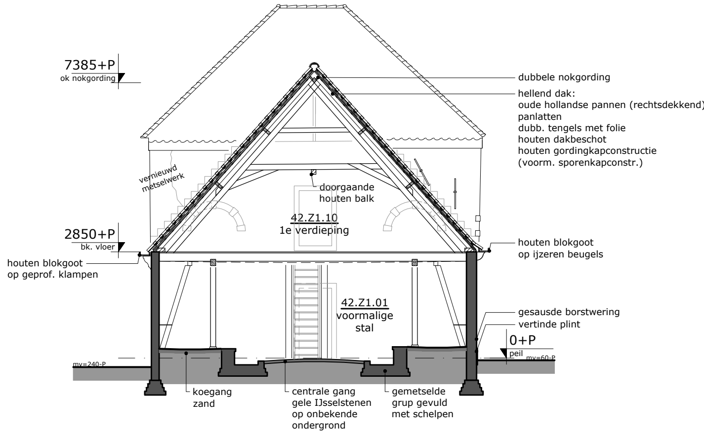
DOORSNEDE E bouwdeel 42_Z1 doorsnede van hoofdspant
