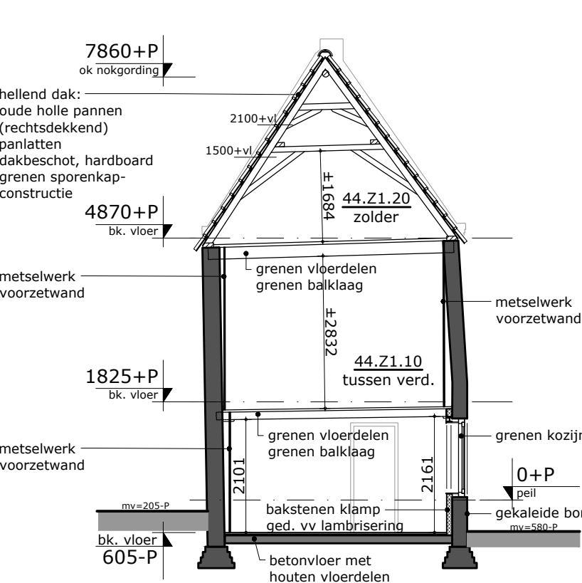
DOORSNEDE B bouwdeel 44_Z1
