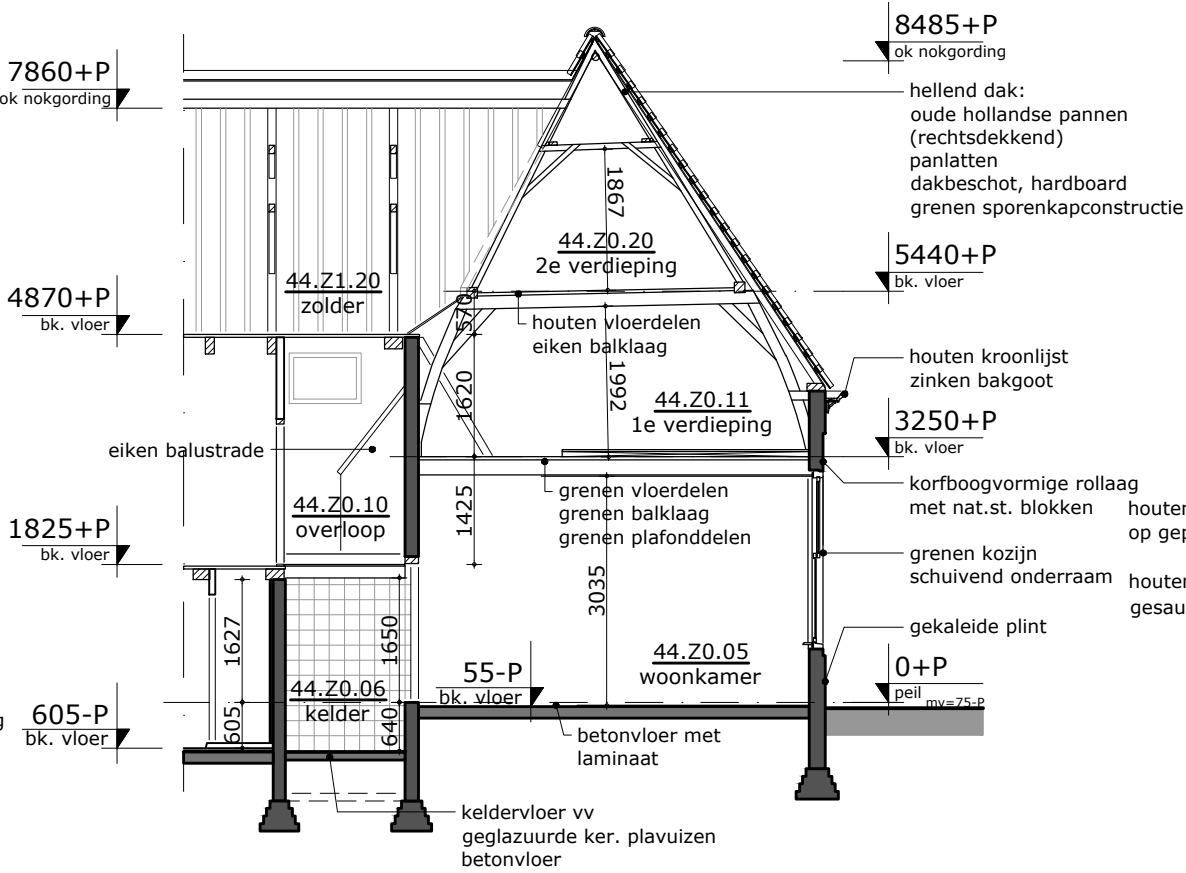
DOORSNEDE C bouwdeel 44_Z0
