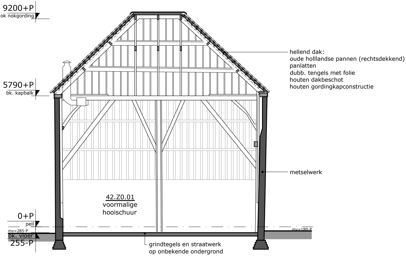
DOORSNEDE F bouwdeel 42_Z0
