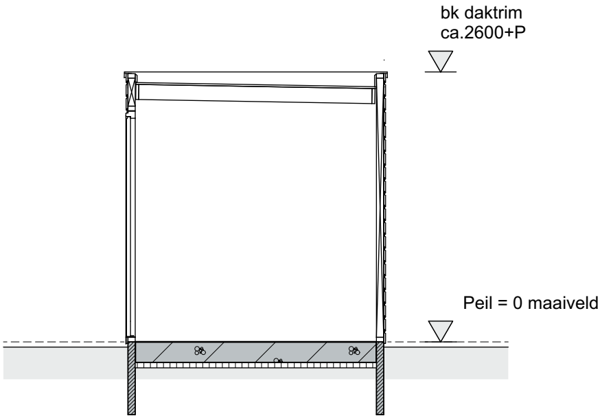
doorsnede
