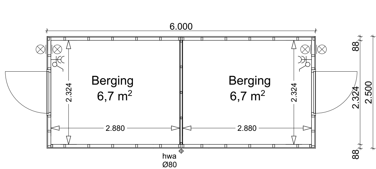
plattegrond
