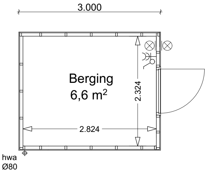
plattegrond
