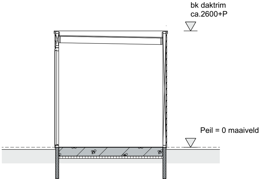
doorsnede
