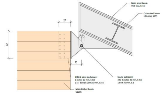
Section A-A S 1:20
