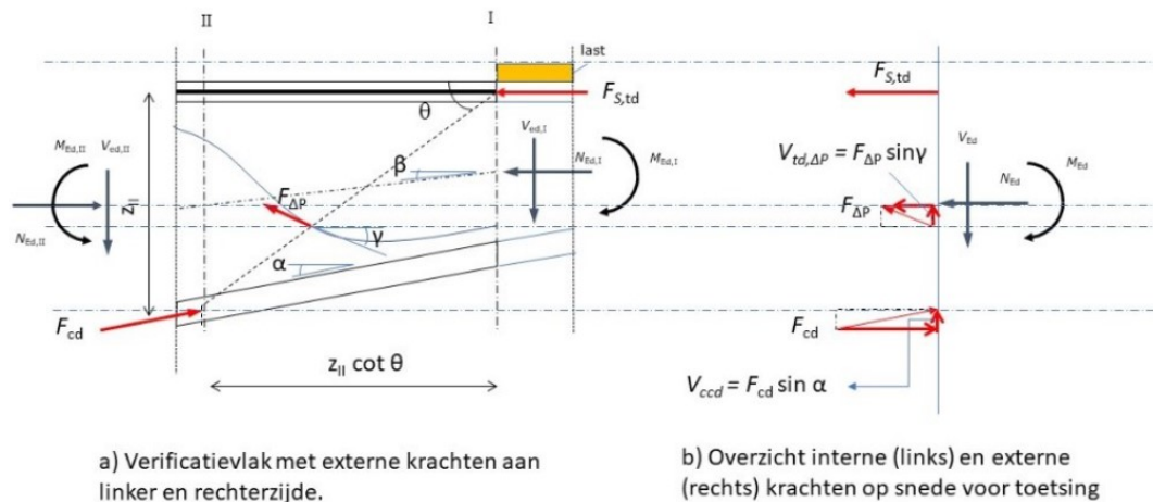
Figuur C4: Snedekrachten bij verlopende ondervloer
