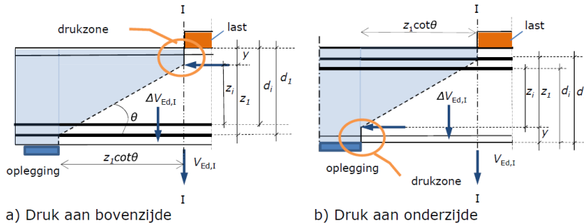
Figuur C3: Verificatievlak bij afschuifbuigbreuk
