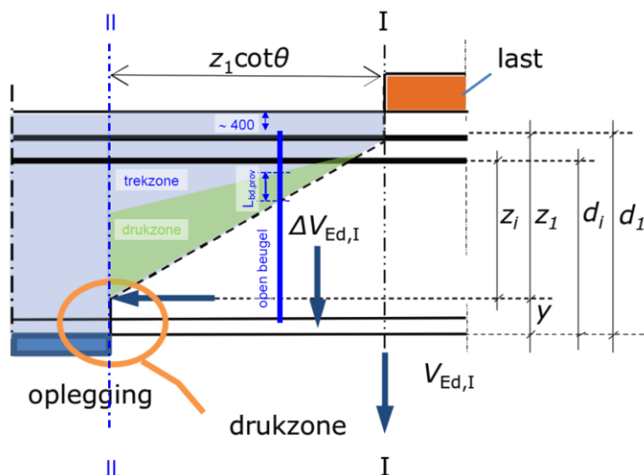
Figuur C2: Drukzone voor bijdrage verticale wapening.
