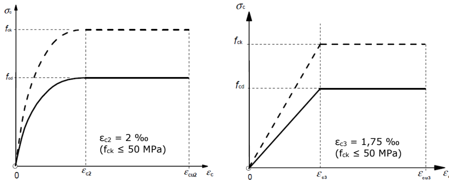
Figuur B2: Parabool-rechthoekig (links) en bi-lineair spanning rekdiagram (rechts)
