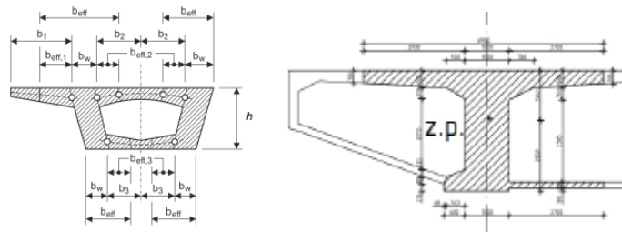
Figuur B1: Effectieve buigdoorsnede.
