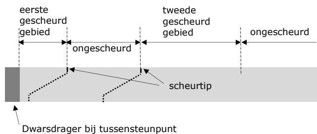
Figuur C1: Verificatievlakken bij overgang gescheurd-ongescheurd gebied.
