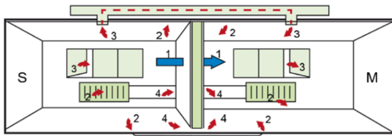
Figuur Fout! Geen tekst met de opgegeven stijl in het document..1 Illustratie geluidoverdracht via verschillende constructies
