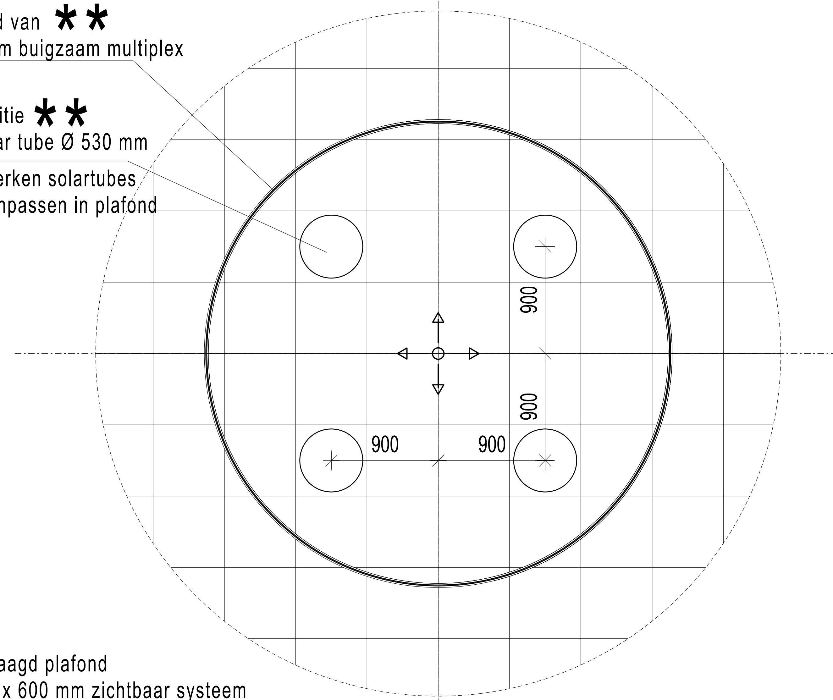
Plafondplan 1:20
