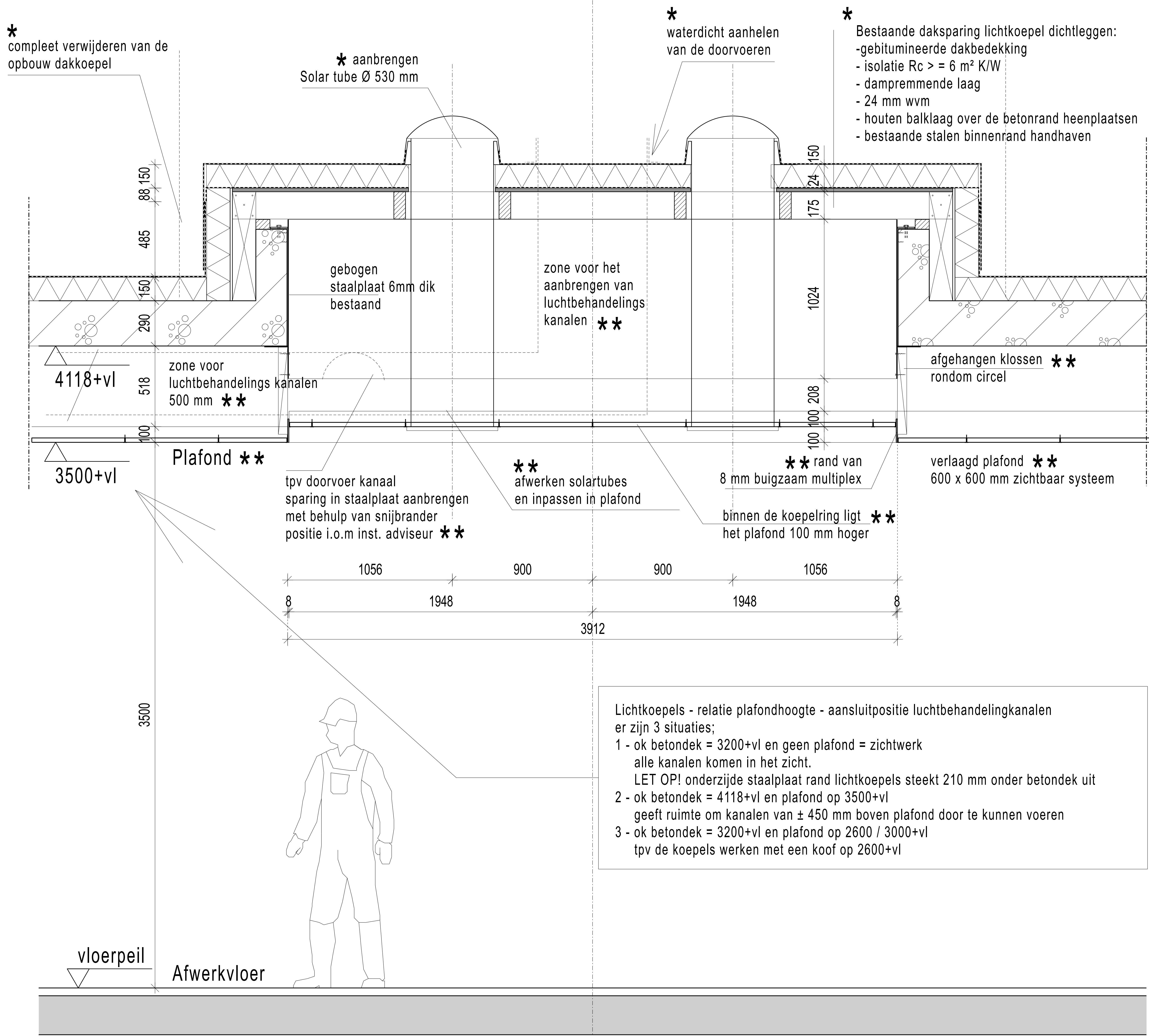
Doorsnede 1:10
