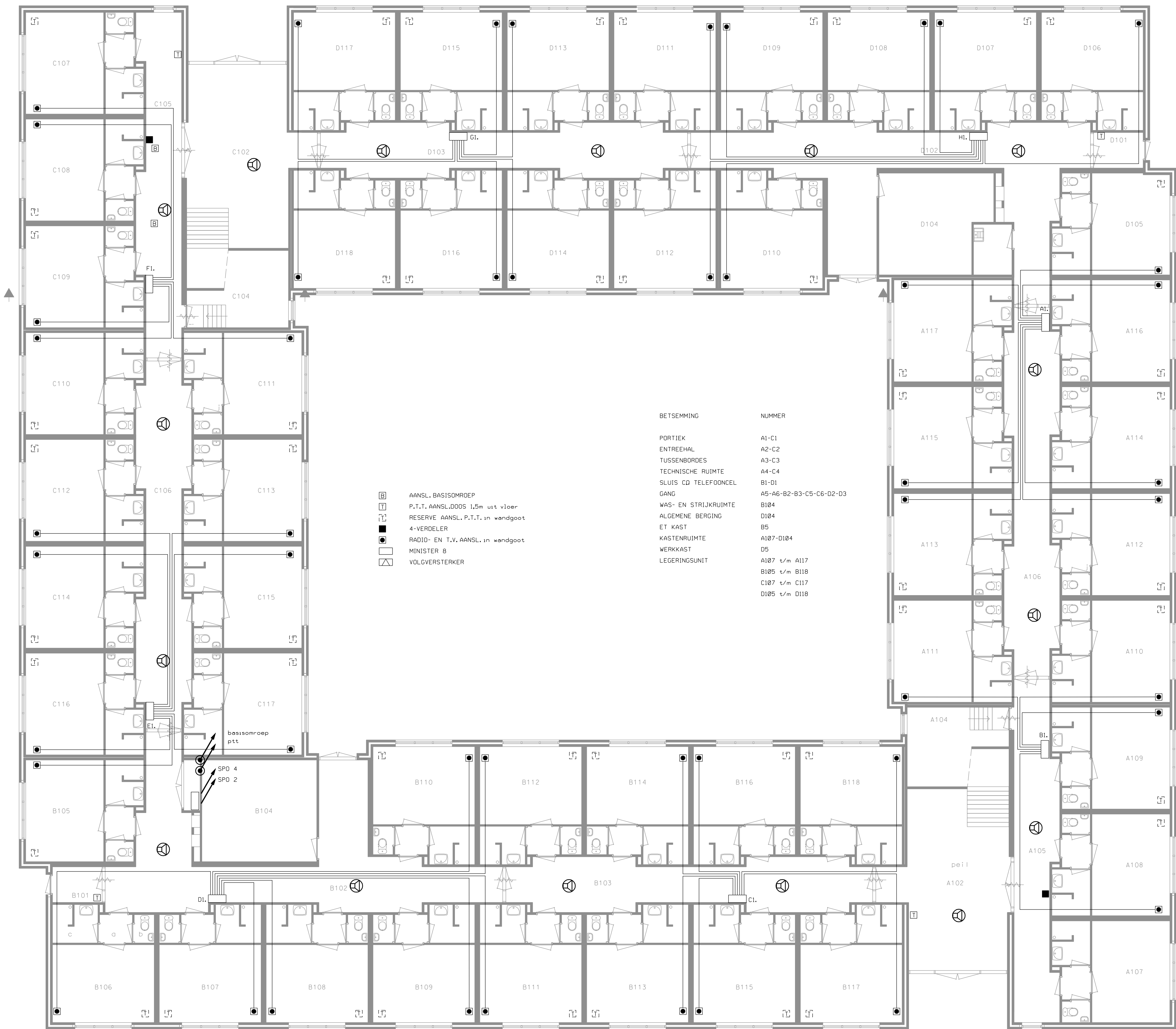
FIG.10. RADIO-, T.V.- EN BASISOMROEPINSTALLATIE. BEGANE GROND(schaal 1:100)
