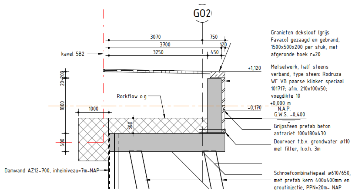
Figuur 1: Indicatie principe doorsnede halfhoge kademuur
