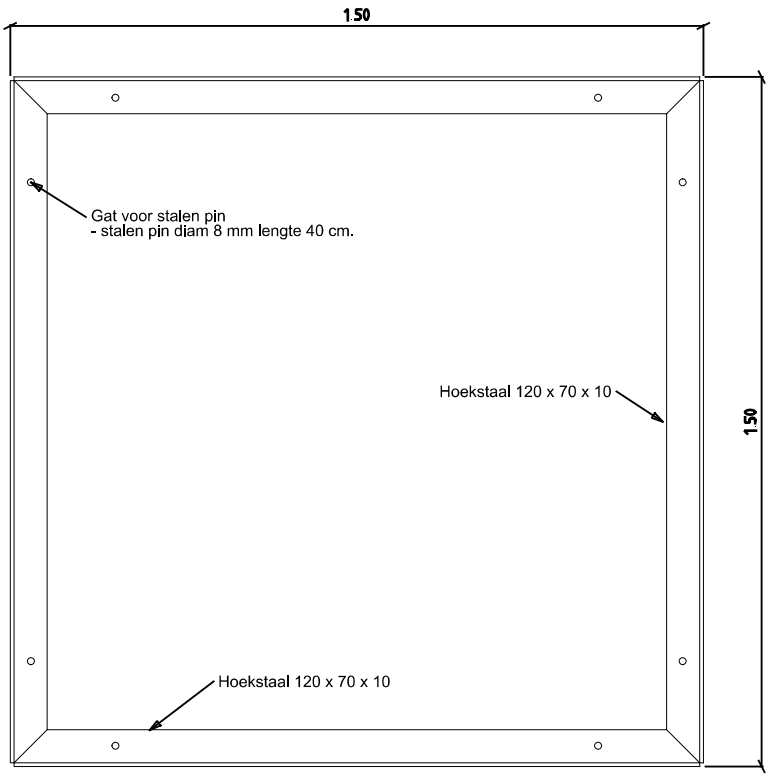
Hoekstaal 120 x 70 x 10 mm Frame
