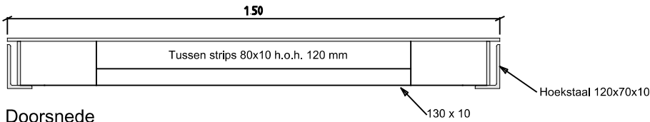
Doorsnede
