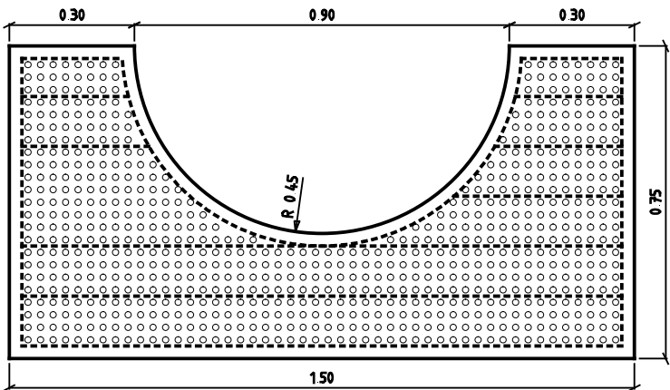
CorTenstalen plaat dik 10 mm Bovenaanzicht
