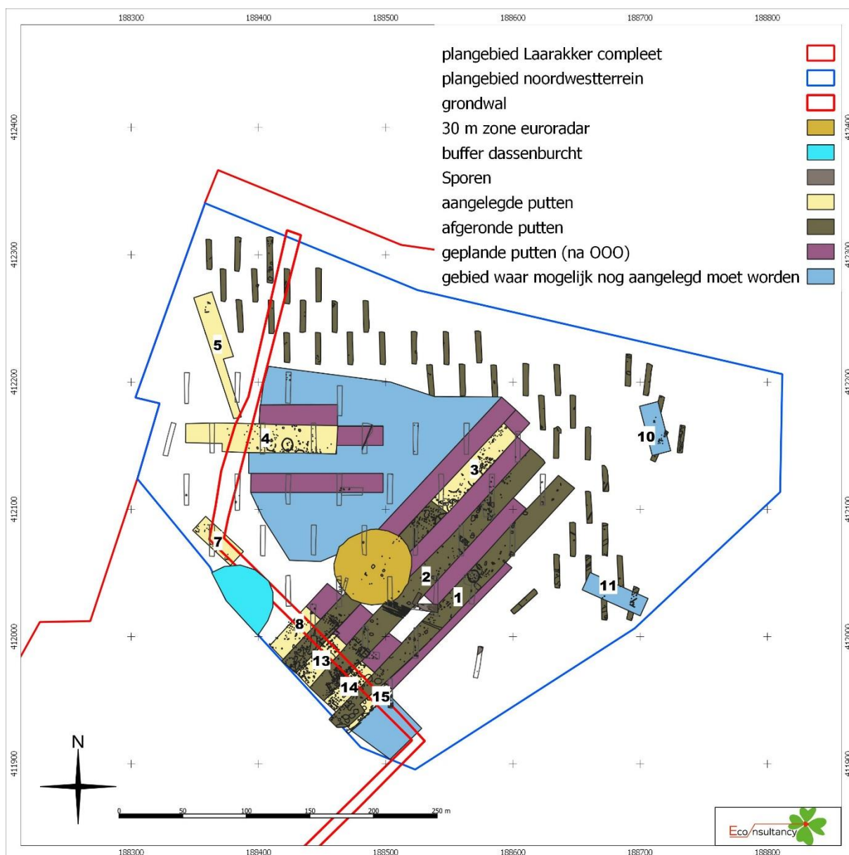
Figuur 1 Puttenplan
