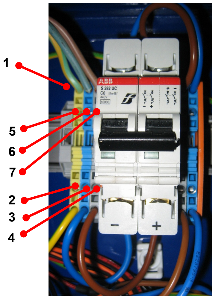
figuur 37 Aansluitblok in de master-monitor
