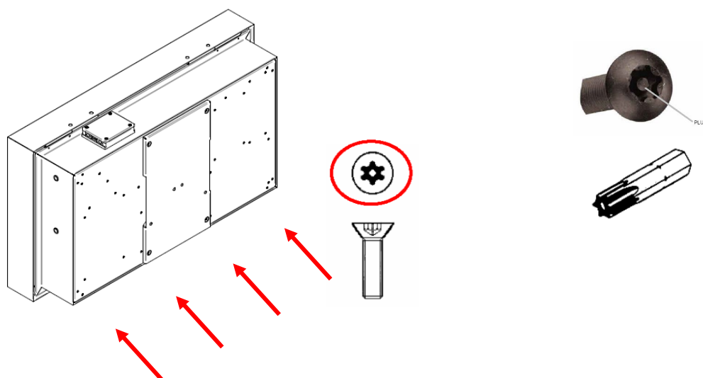
figuur 32 Positie van de schroeven en type schroeven en schroevendraaier
