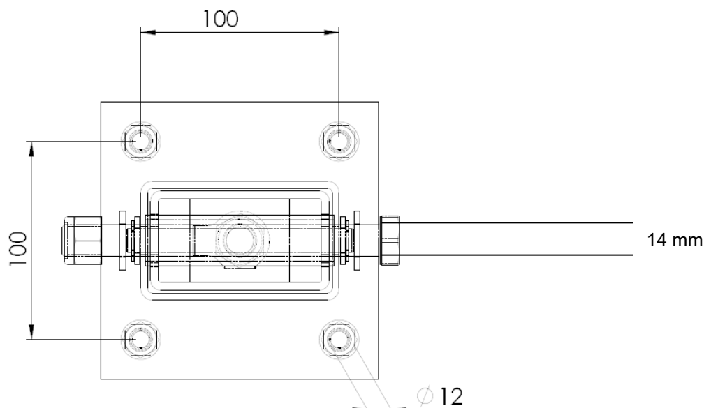
figuur 16 Detail instelbare pendel
