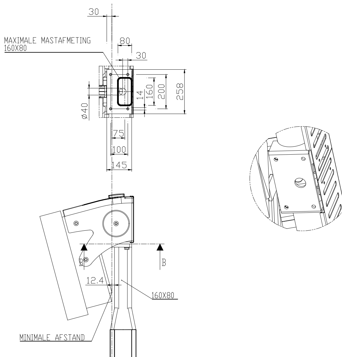
figuur 25 Doorsnede tekening van een enkelzijdig presentatiemiddel op een mast.
