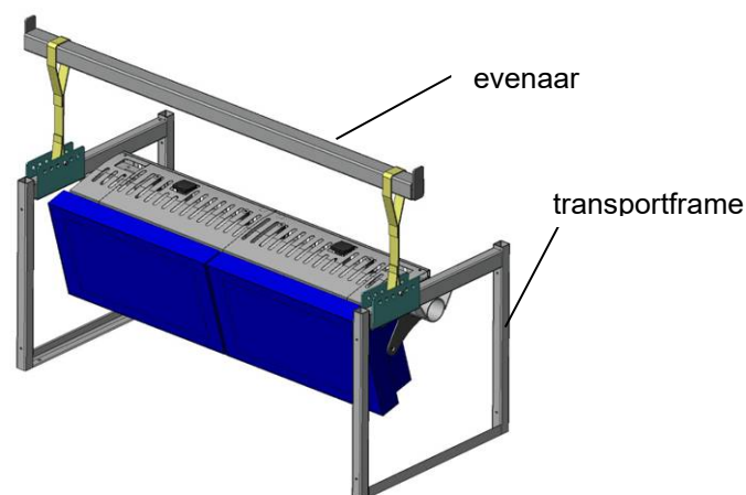
figuur 23 Enkelzijdig presentatiemiddel hijsen met evenaar
