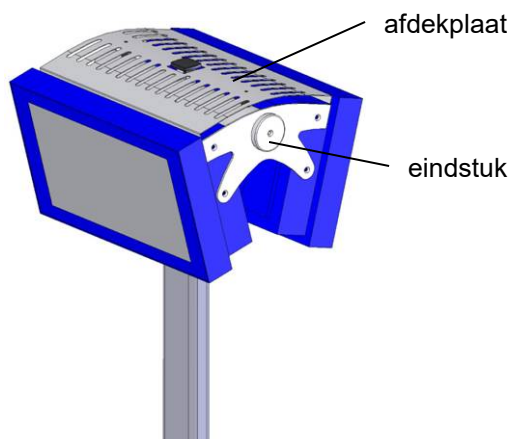
figuur 28 Dubbelzijdige TB-1 op mast.
