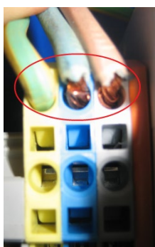
figuur 40 Aansluitmethode: NIET ACCEPTABEL
