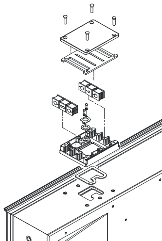
figuur 34 Opbouw kabelinvoerdoos
