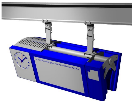
figuur 20 Montage van de afdekplaten
