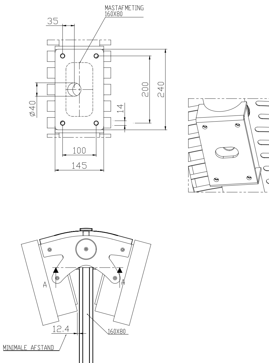
figuur 26 Doorsnede tekening van een dubbelzijdige TB-xx op een mast.
