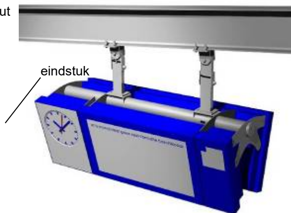
figuur 19 Montage van de eindstukken
