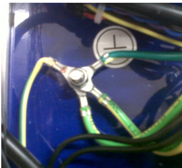
figuur 41 Aansluitpunt aarddraad in een 32" module bij de TB-xx wandbevestiging
