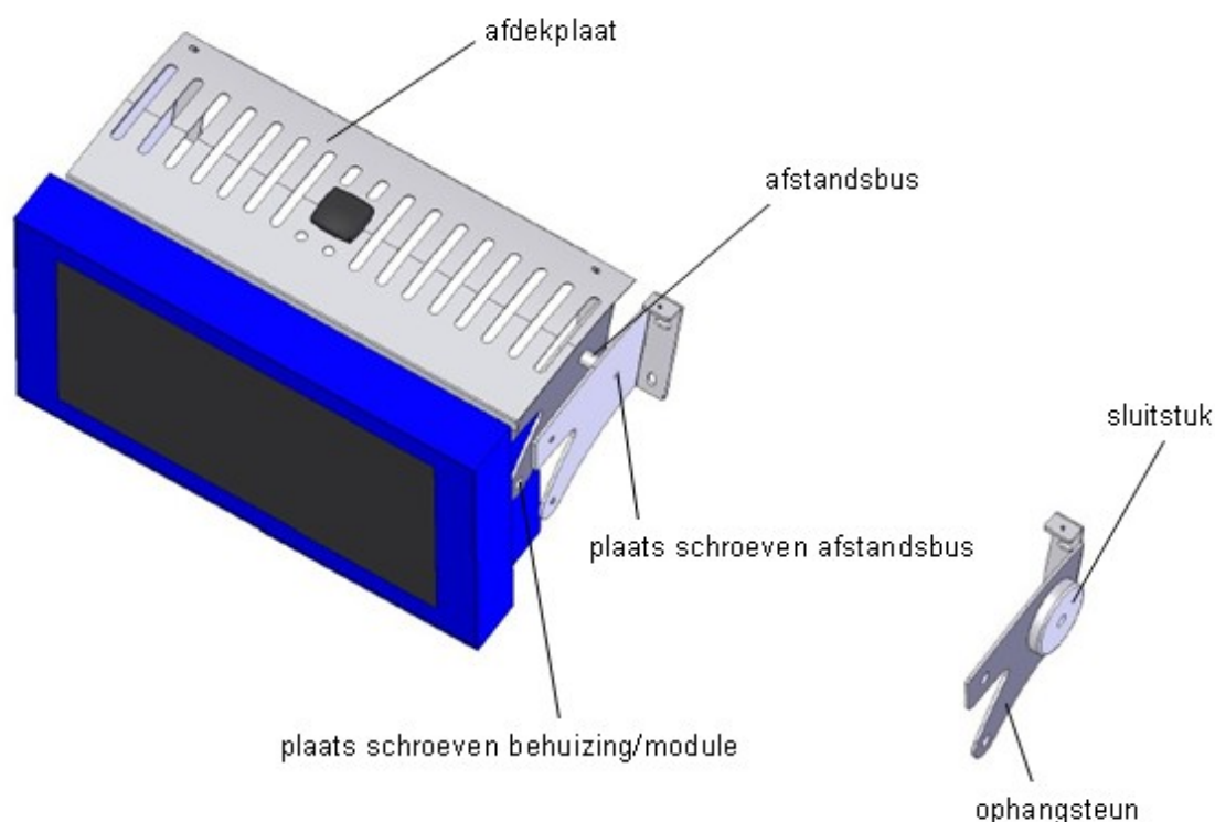
figuur 30 Montage presentatiemiddel type wandbevestiging
