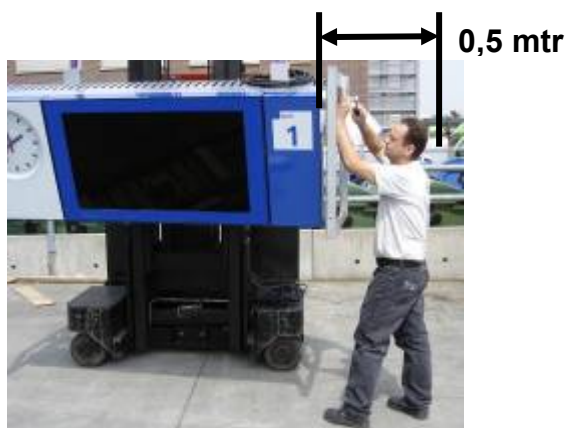
figuur 12 Demontage van de transportsteun
