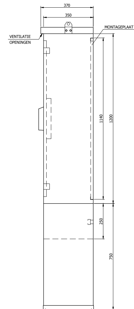
ZIJAAANZICHT RECHTS
