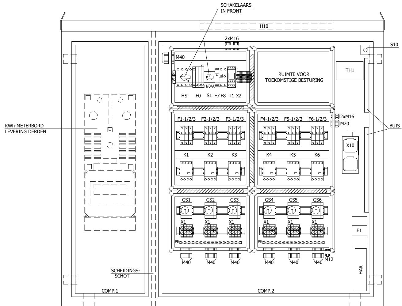
VOORAANZICHT (ZONDER DEUREN EN SOKKEL)
