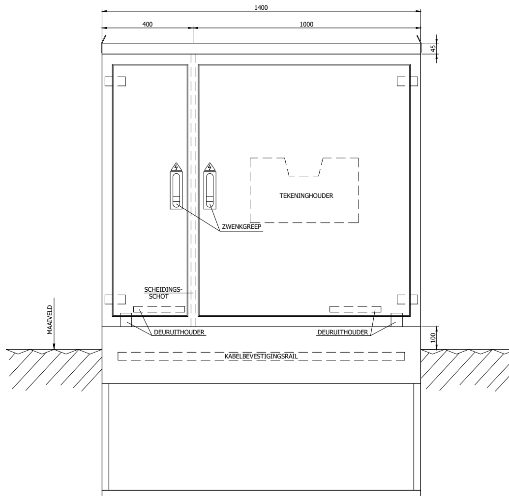
VOORAANZICHT
