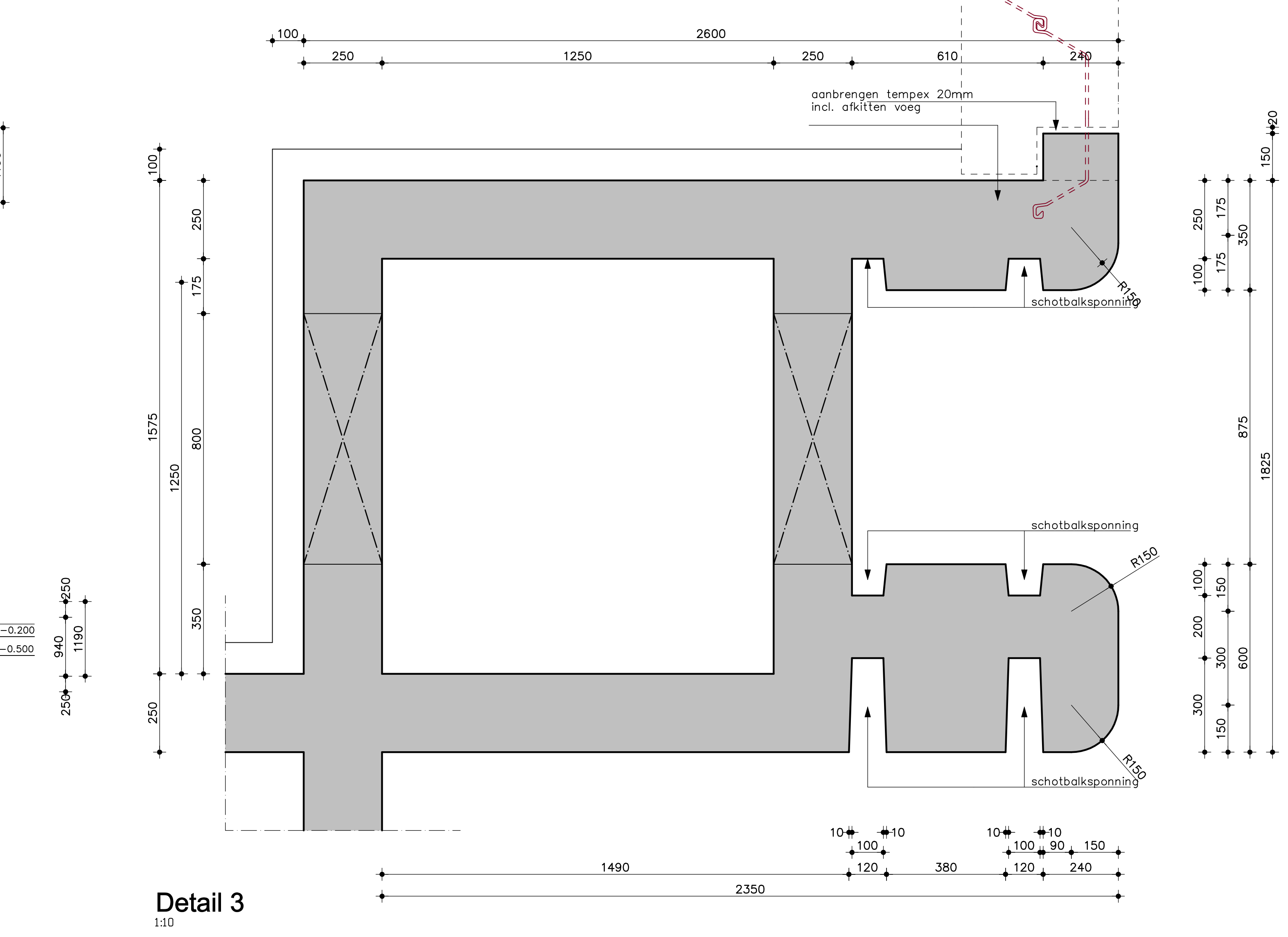
Algemeen detail aansluiting damwand L603 met deksloof
