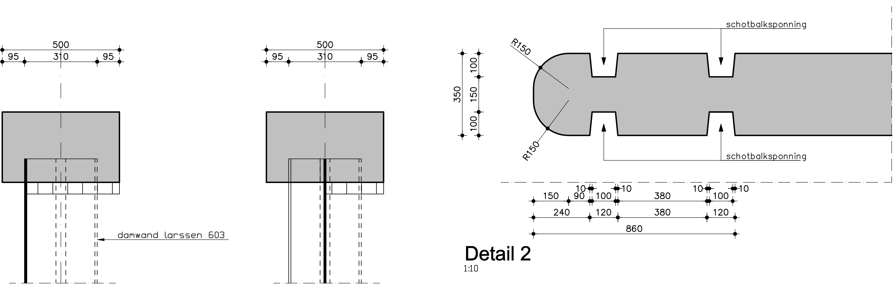
Algemeen detail aansluiting damwand L603 met deksloof
