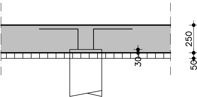
Algemeen paalkopdetail 1:20
