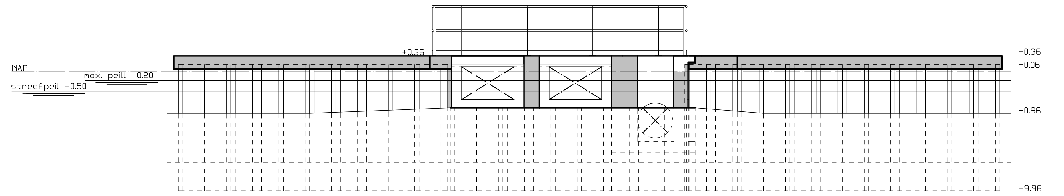
Aanzicht uitstroom 1:50
