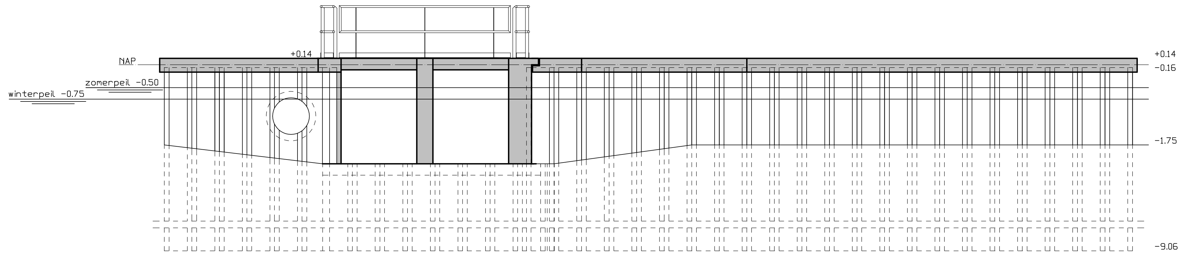
Aanzicht instroom 1:50
