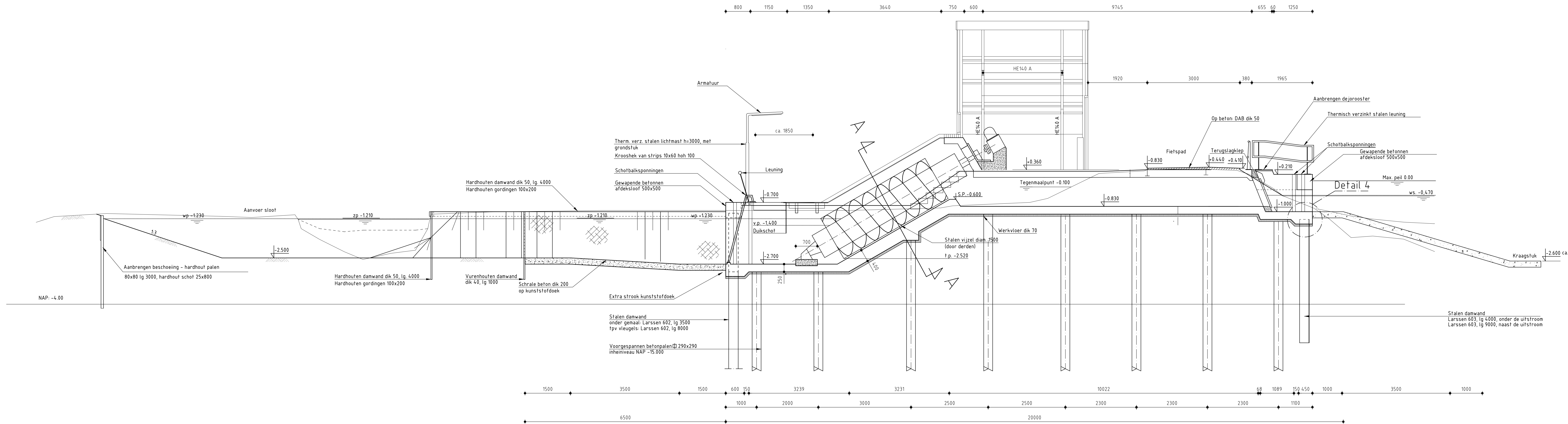
Dwarsdoorsnede schaal 1:50
