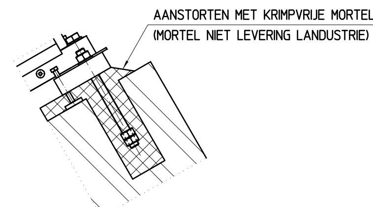
DETAIL ANKERS FUNDATIE AANDRIJVING NET OP SCHAAL
