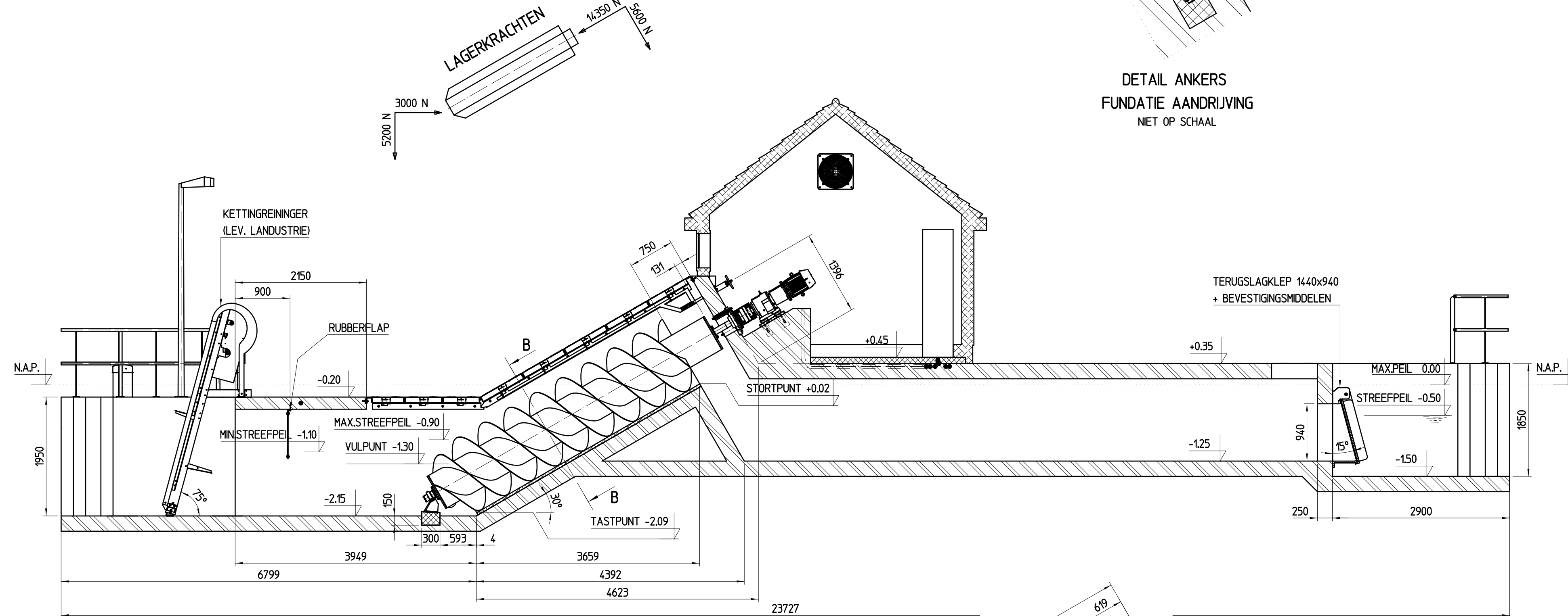
DOORSNEDE A-A
