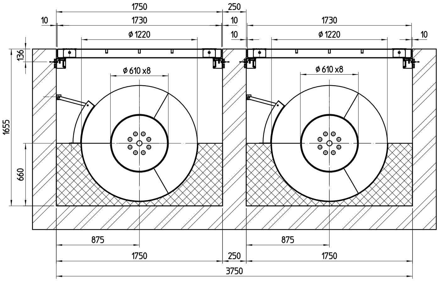
DOORSNEDE B-B SCHAAL 1:25
