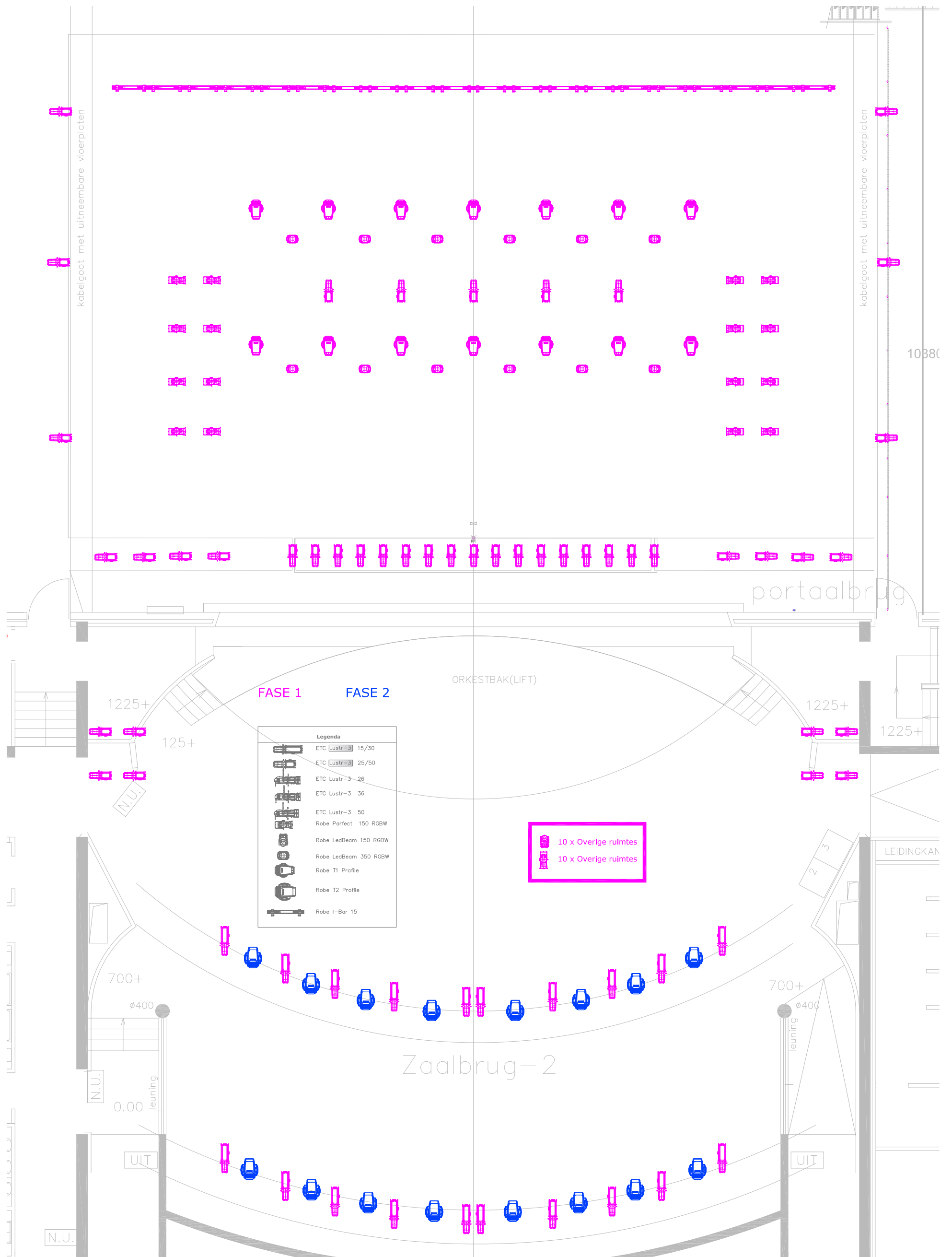
A3, 1:100, Goudse Schouwburg, Lichtplan GZ LED
