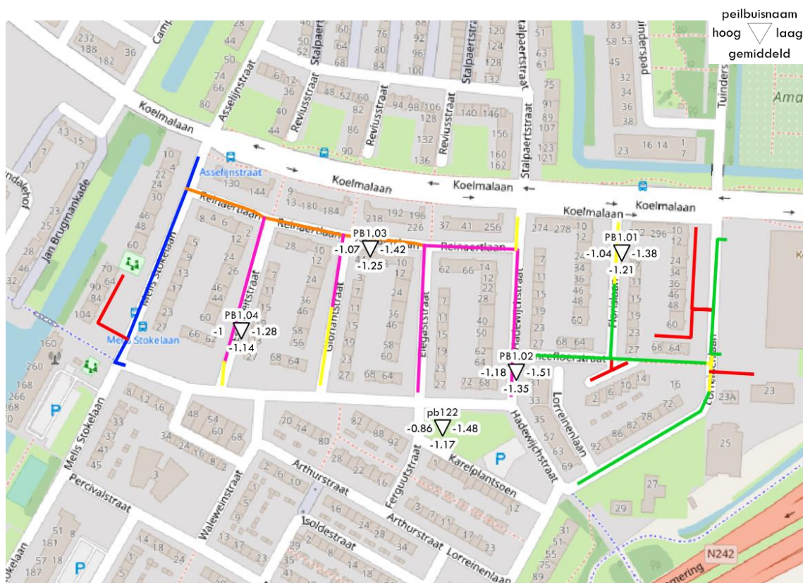
figuur 6 - grondwaterstand t.o.v. NAP per geanalyseerde peilbuis (wit = freatisch/watervoerende laag 1, rood = watervoerende laag 3)
