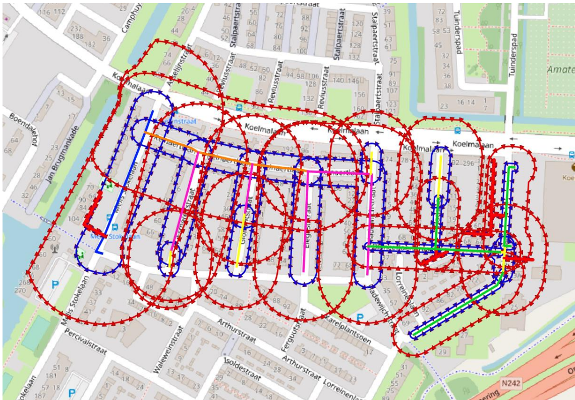
figuur 5 – reikwijdte bemaling, grootste reikwijdte per watervoerende laag is gebruikt voor deze figuur (blauw=prognose onder normale omstandigheden, rood=extreem bij een natuurlijk lage grondwaterstand/droge periode)
