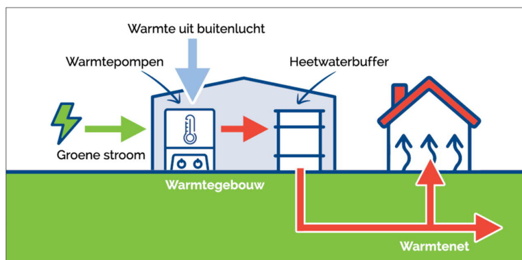
Concept warmtenet Loppersum
