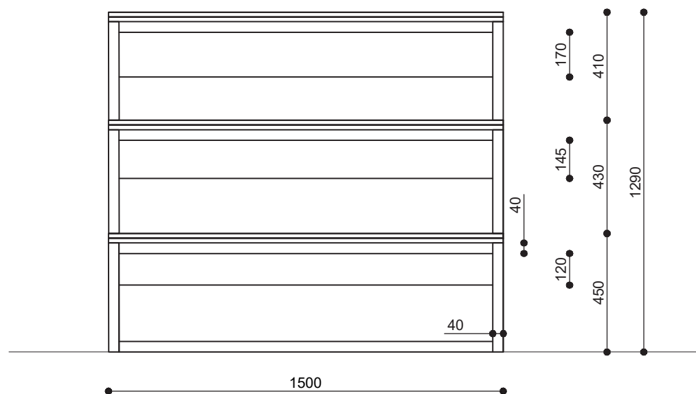
Vooraanzicht
