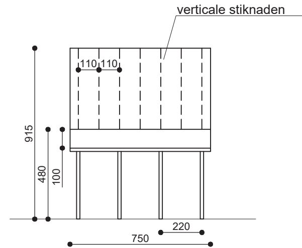
Vooraanzicht
