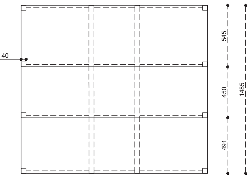
Bovenaazicht met frame
