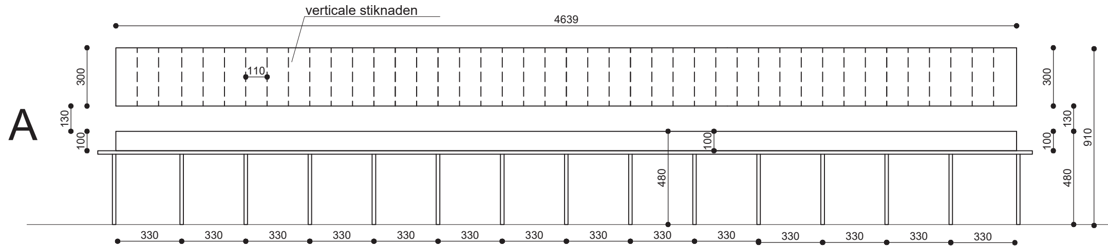
Vooraanzicht
