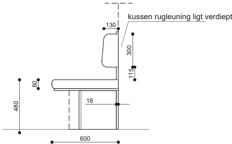
Doorsnede A - ontwerp aangepast meubel
