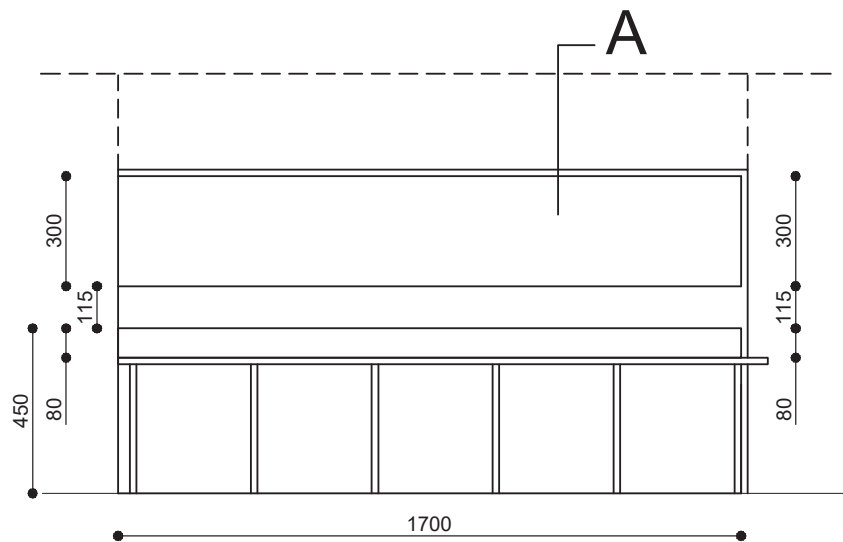
Vooraanzicht - ontwerp aangepast meubel
