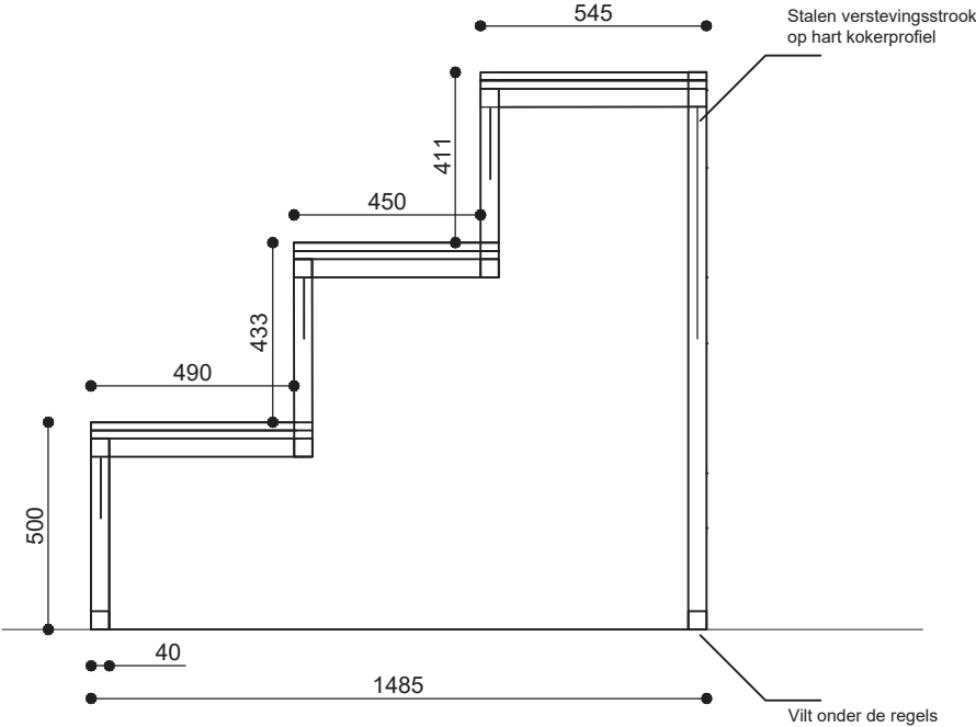
Doorsnede A - verticaal
