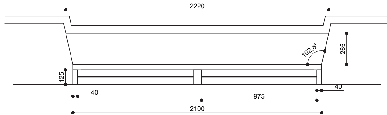
Bovenaanzicht, raamkozijn
