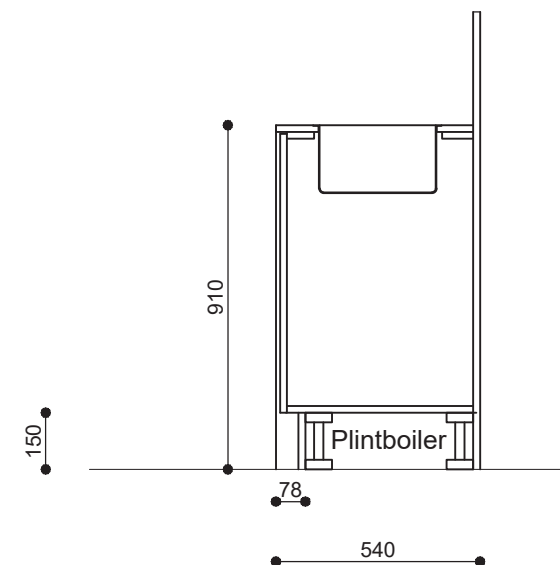
Doorsnede A
