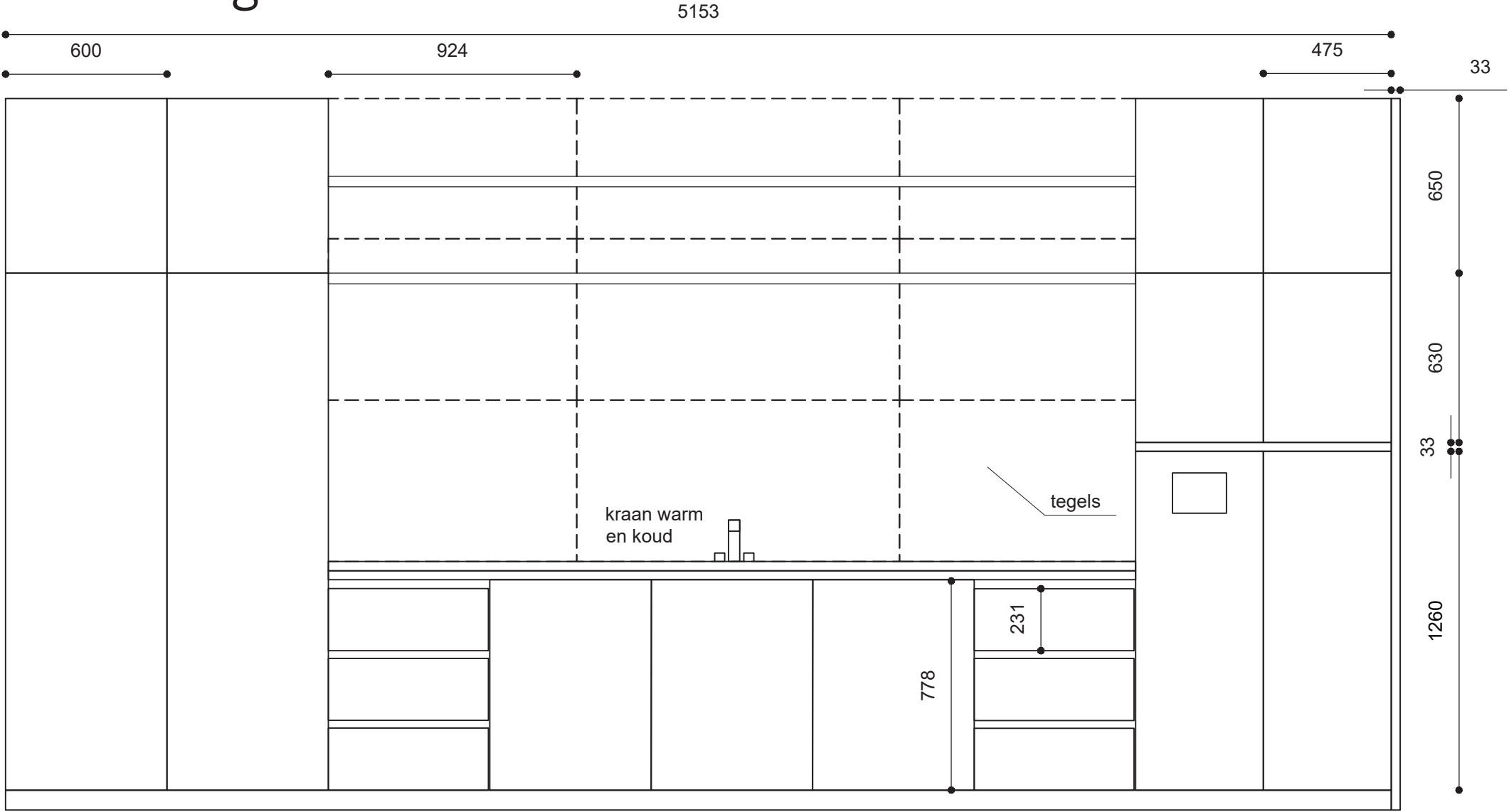
Vooraanzicht
