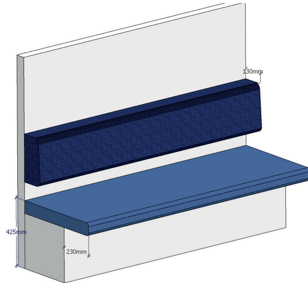
Bestaand meubel
