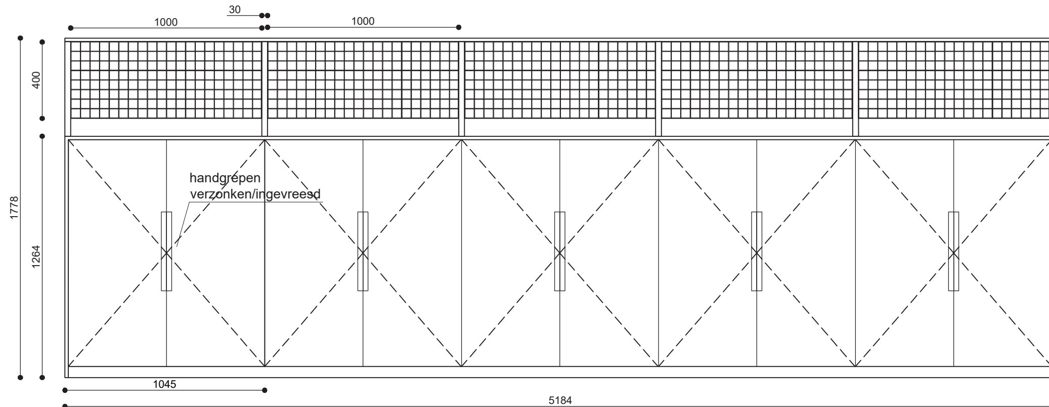
vooraanzicht
