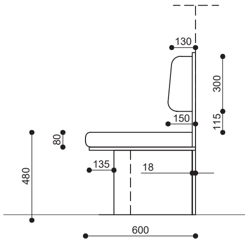
Zijaanzicht - ontwerp aangepast meubel
