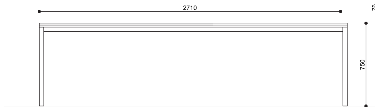
Vooraanzicht
