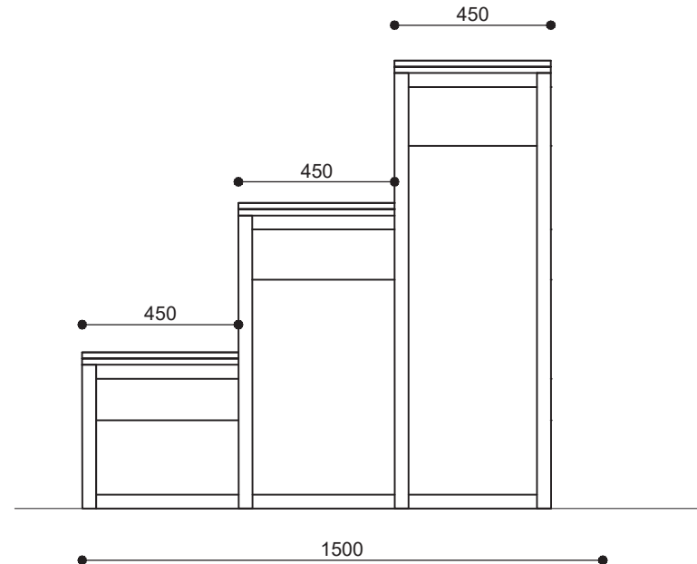
Zijaanzicht
