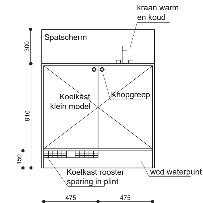
Vooraanzicht
