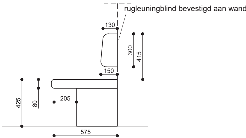
Zijaanzicht - huidige situatie
