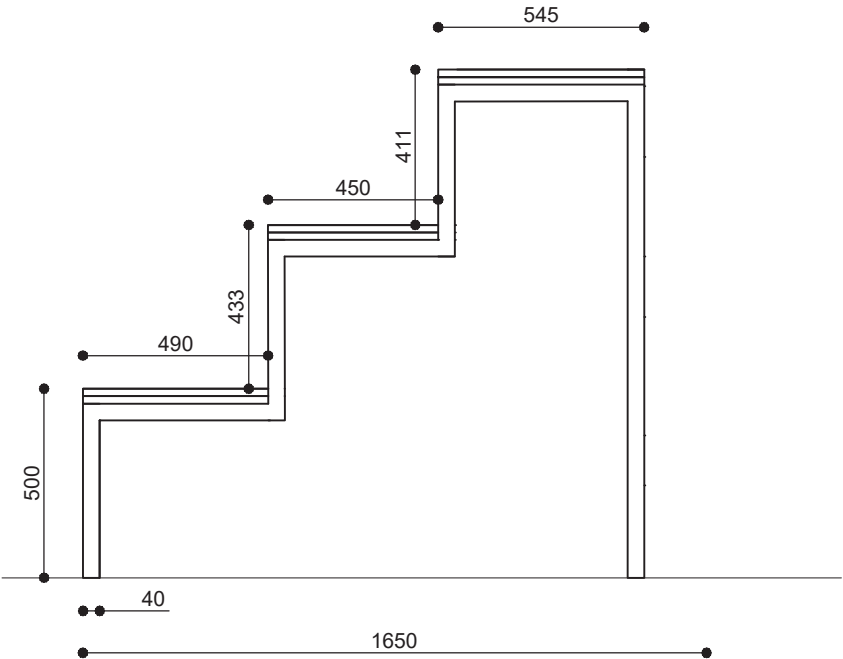
Zij aanzicht
