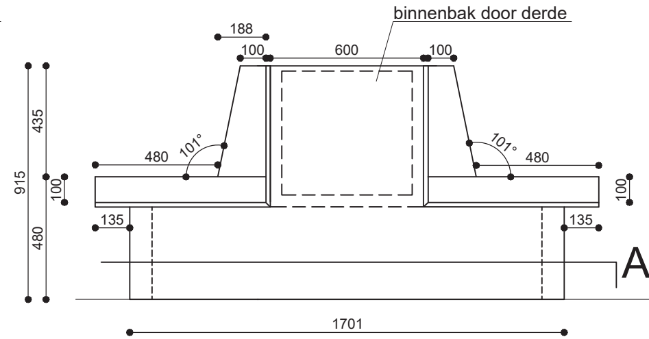
Zijaanzicht
