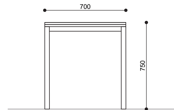
Zijaanzicht
