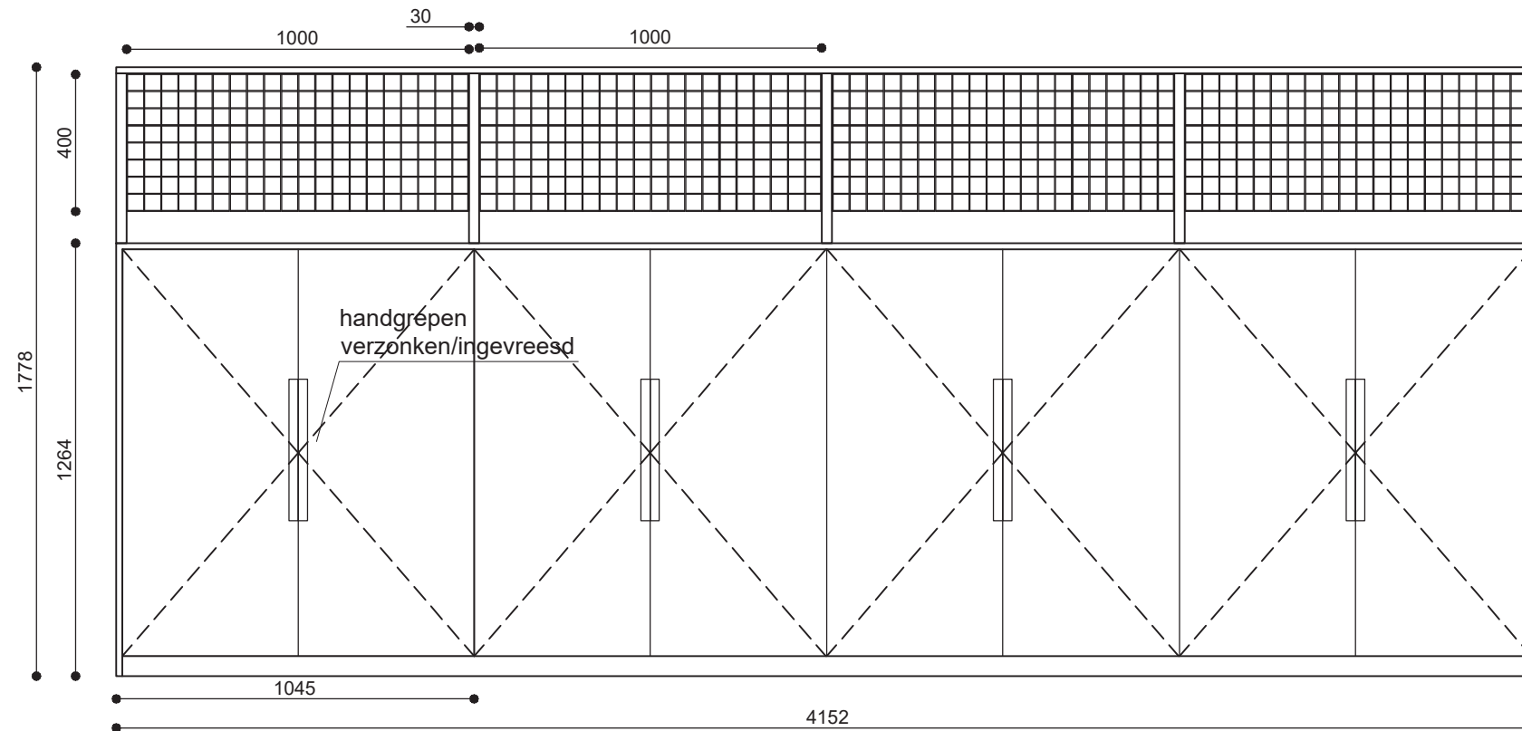
vooraanzicht
