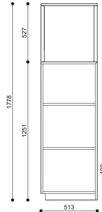
doorsnede
