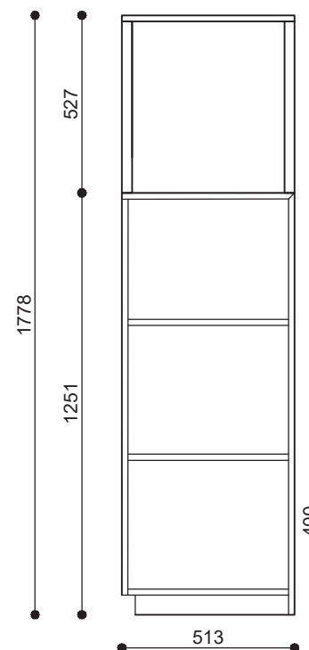
doorsnede
