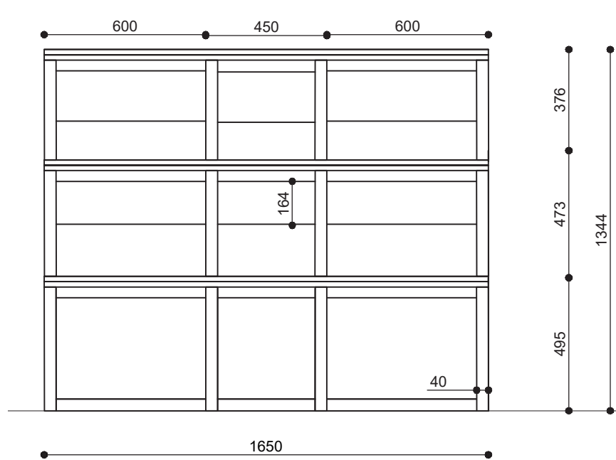
/ooraanzicht
