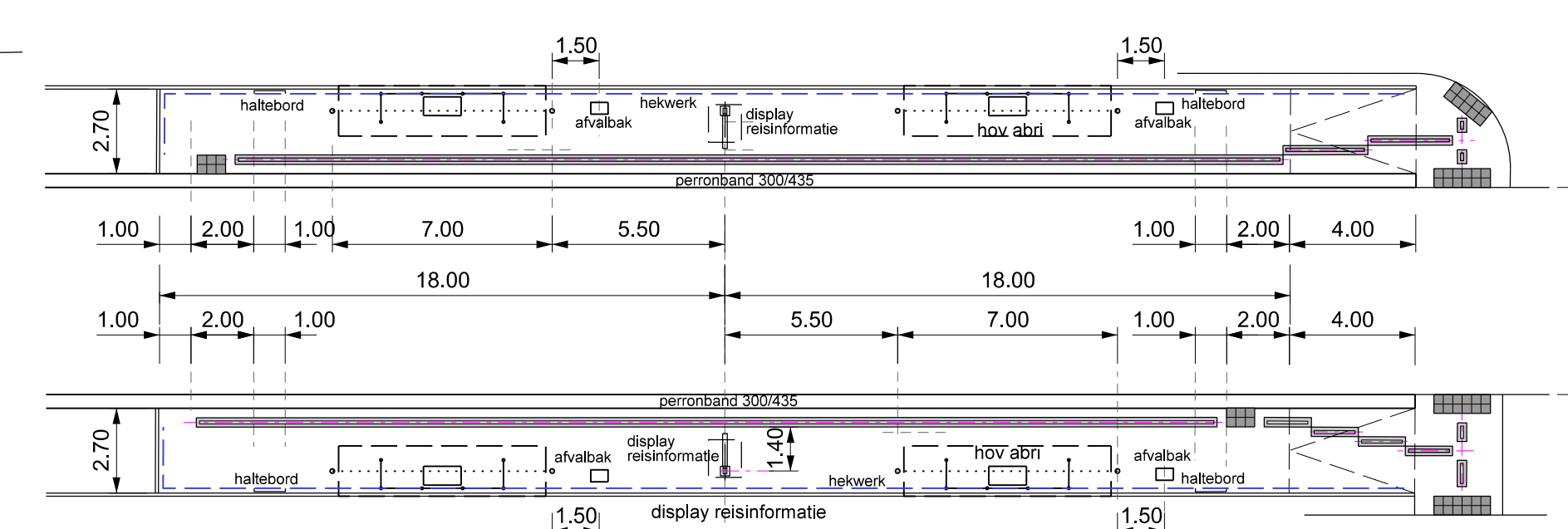
Detail halte Estafettebaan Schaal 1:200
